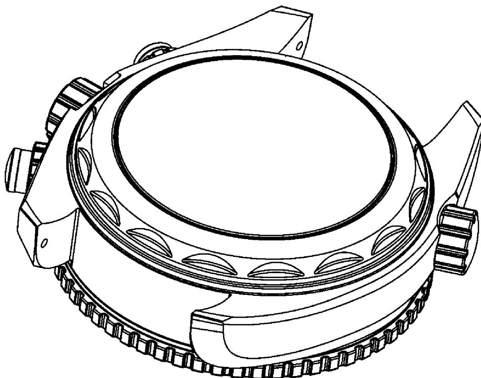
【立體圖2】
