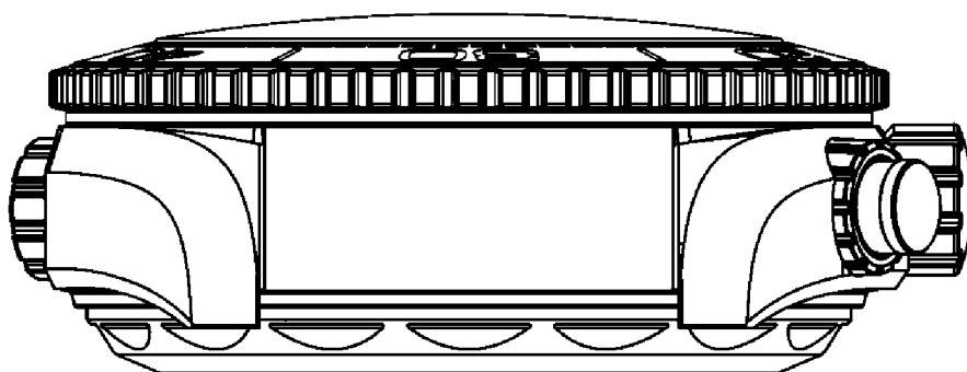
【仰視圖】
