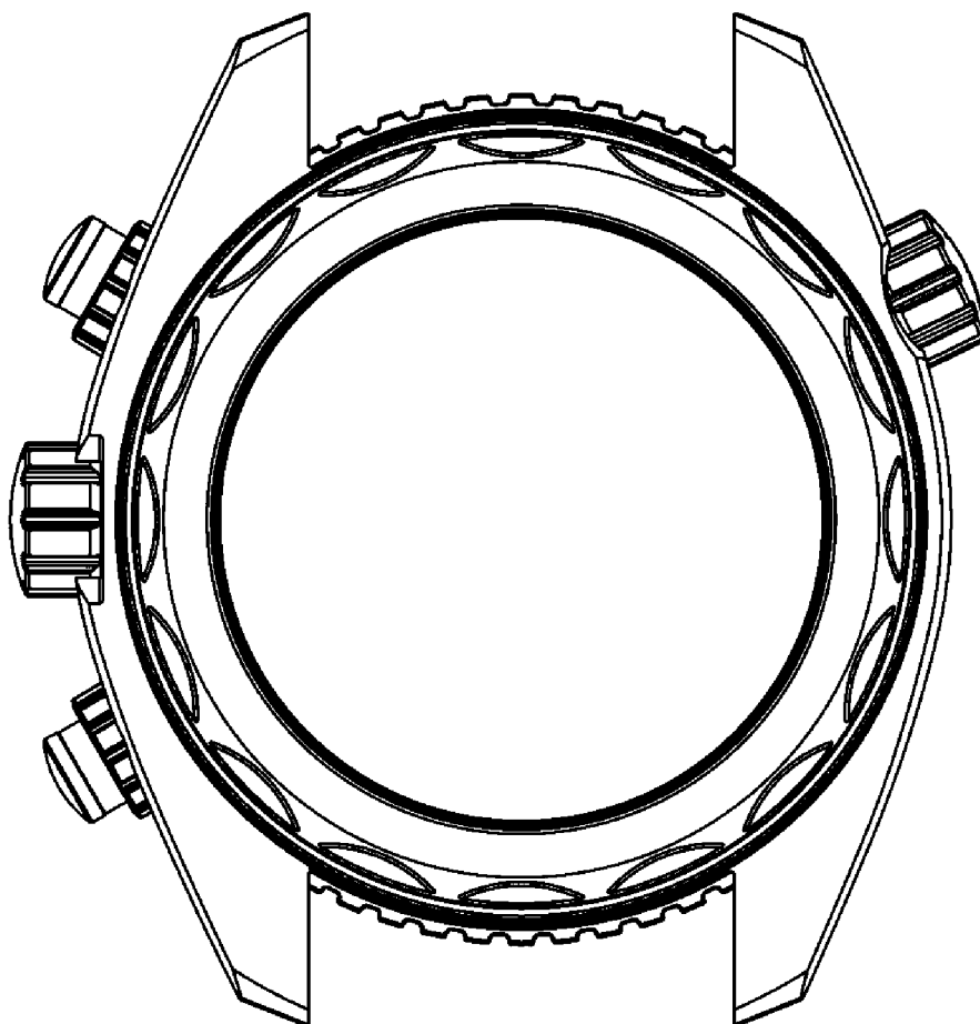
【後視圖】
