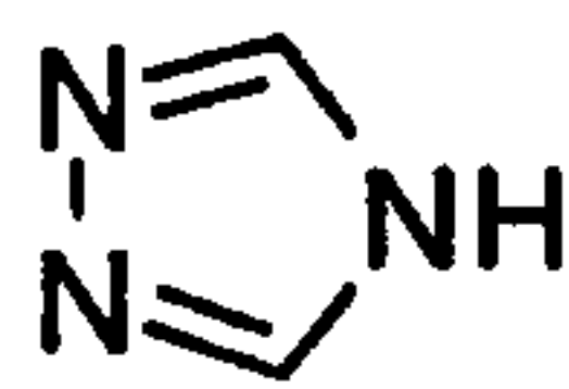
triazole (triazolyl)
