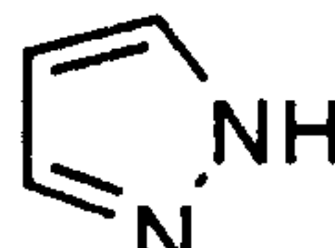
pyrazole (pyrazolyl)
