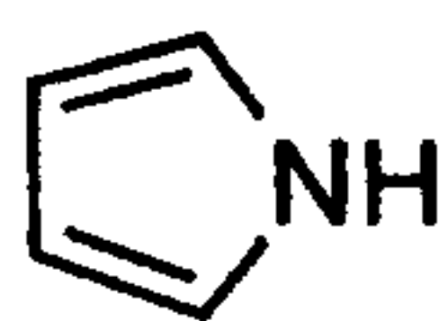
pyrrole (pyrrolyl)
