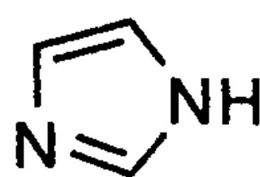
imidazole (imidazolyl)
