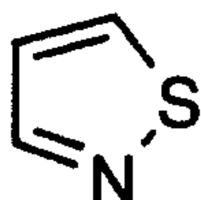
isothiazole (isothiazolyl)
