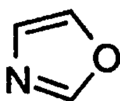
oxazole (oxazolyl)
