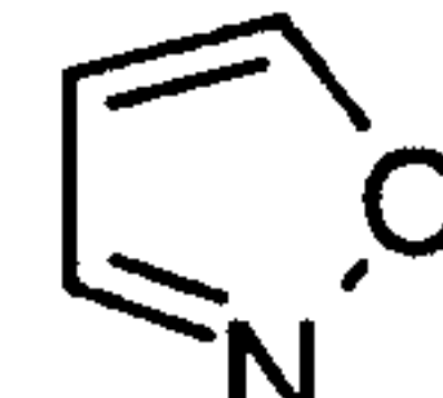
isoxazole (isoxazolyl)
