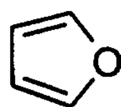
furan (furyl)
