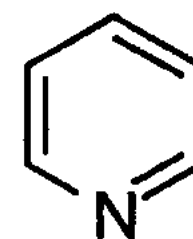
pyridine (pyridinyl)
