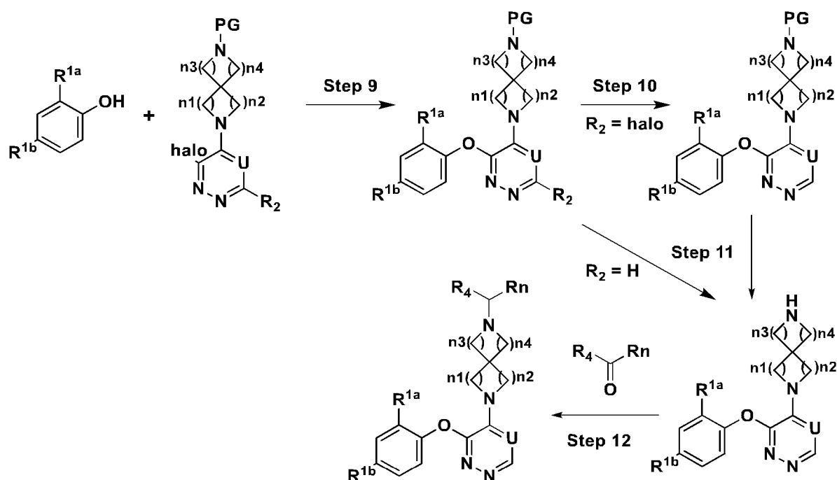
Scheme 2a
