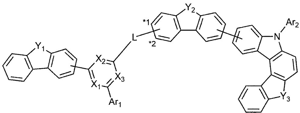
[화학식 3-2]
