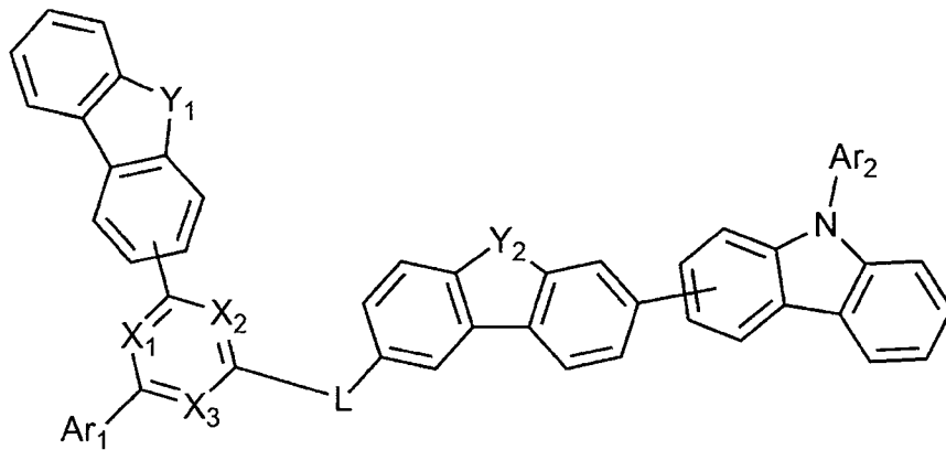
[화학식 1-6]
