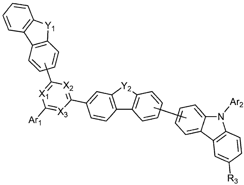
[화학식 1-2]
