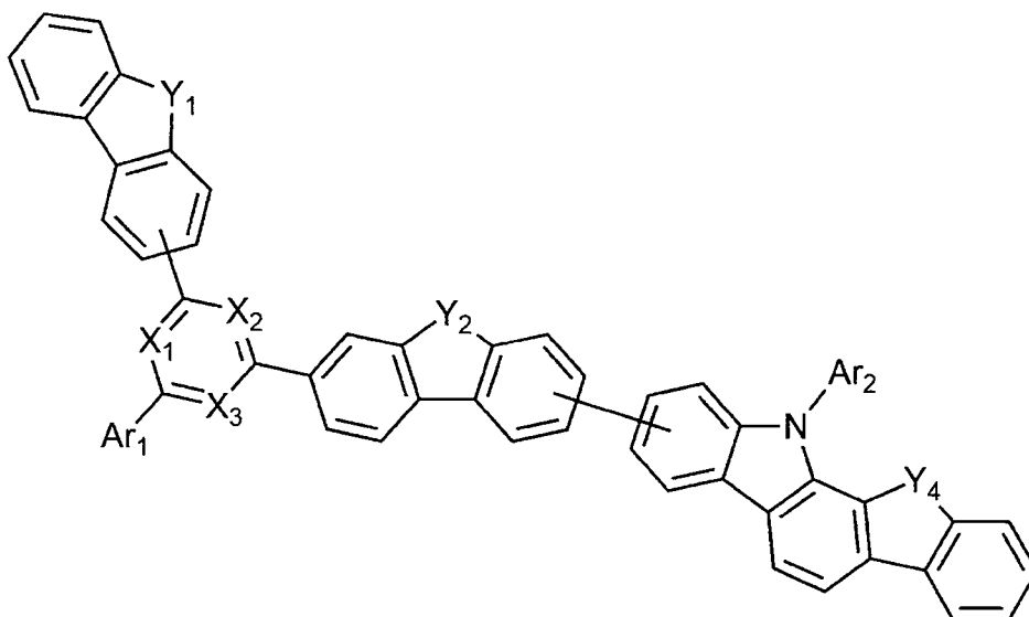
[화학식 1-5]
