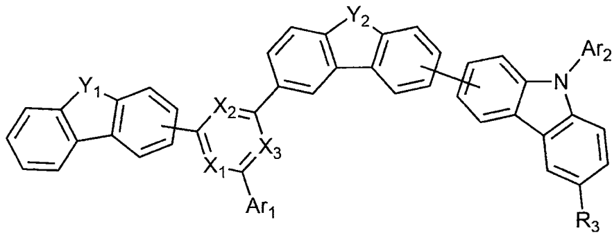
[화학식 1-6]
