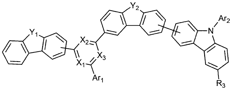
[화학식 1-6]
