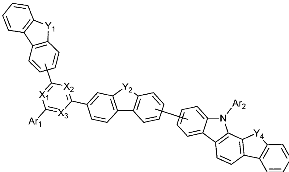
[화학식 1-5]
