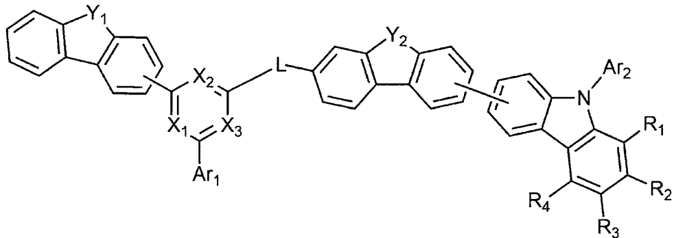
[화학식 1B]
