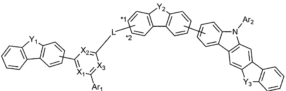
[화학식 3-4]
