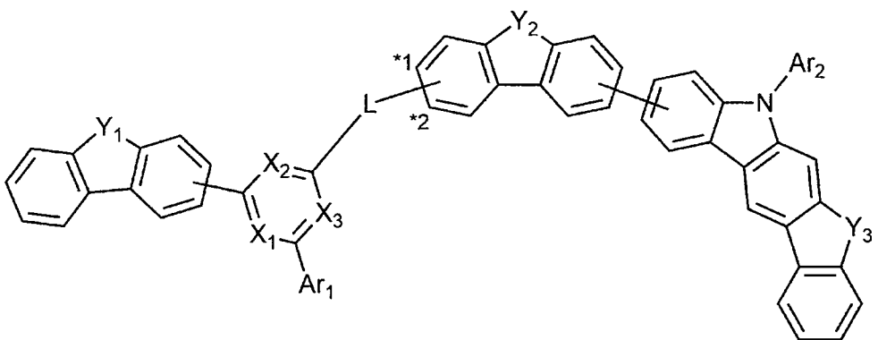
[화학식 3-4]
