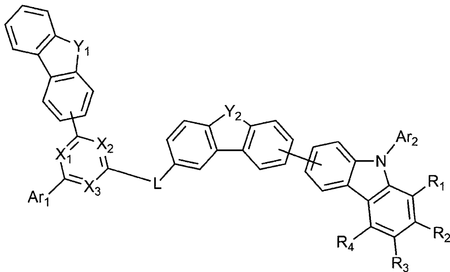
[화학식 1B]
