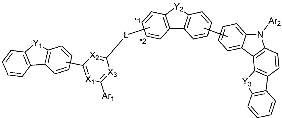
[화학식 3-3]
