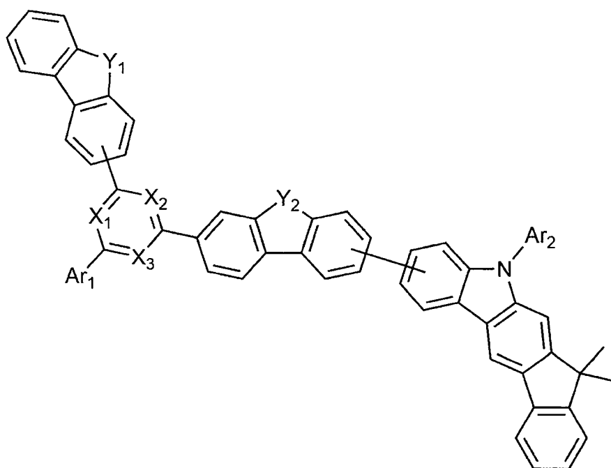
[화학식 1-4]
