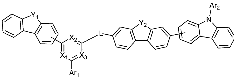
[화학식 1-3]
