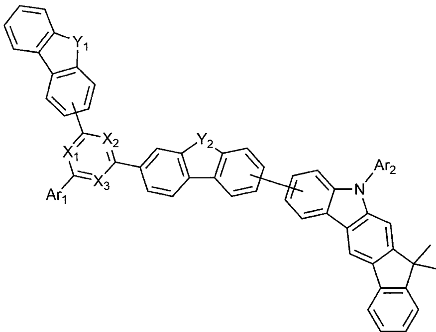
[화학식 1-4]
