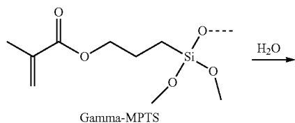
Scheme 12-1.
