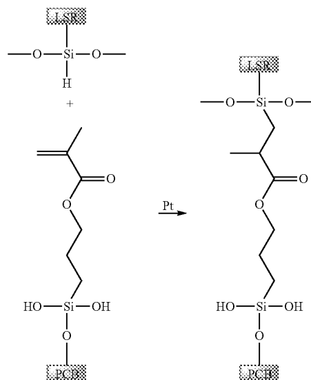
Scheme 12-2.
