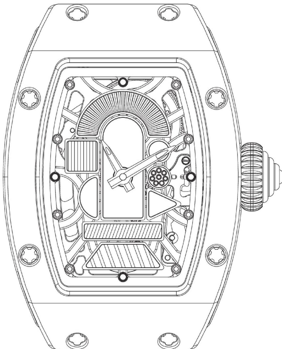
【前視圖】
