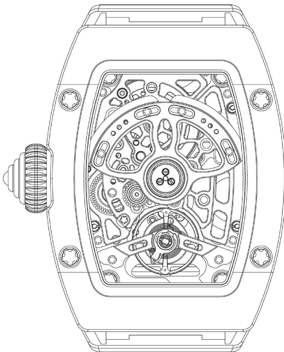
【後視圖】
