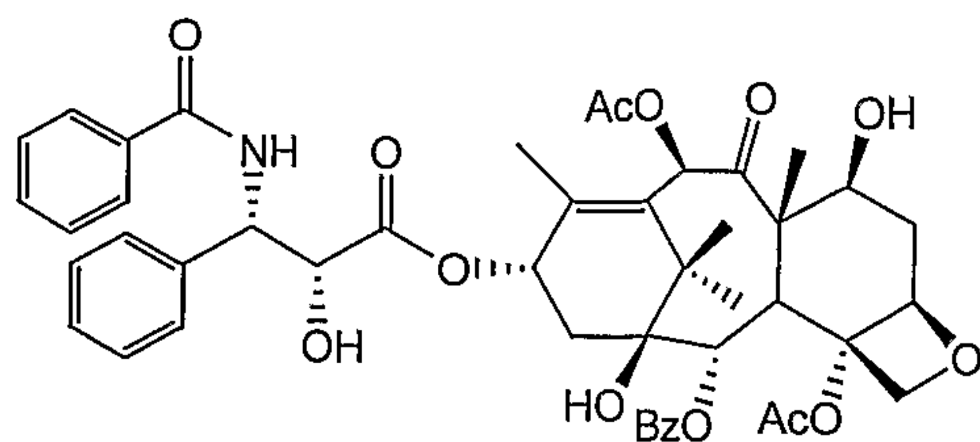
Taxol A (Paclitaxel)
