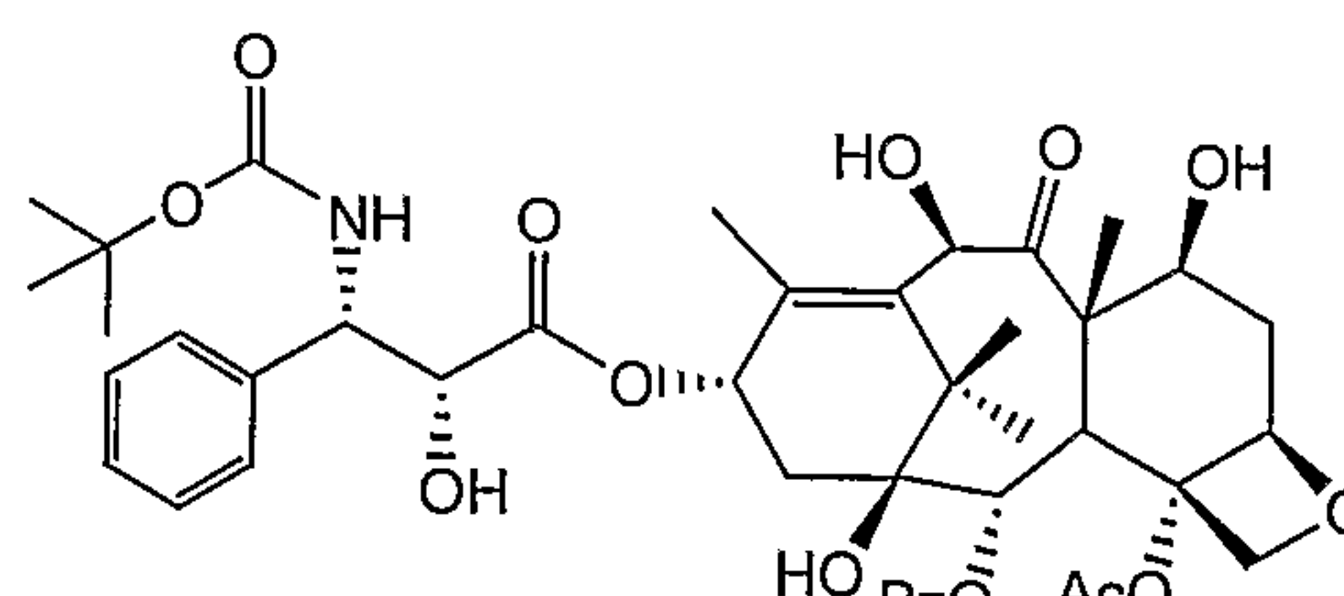
Docetaxel
