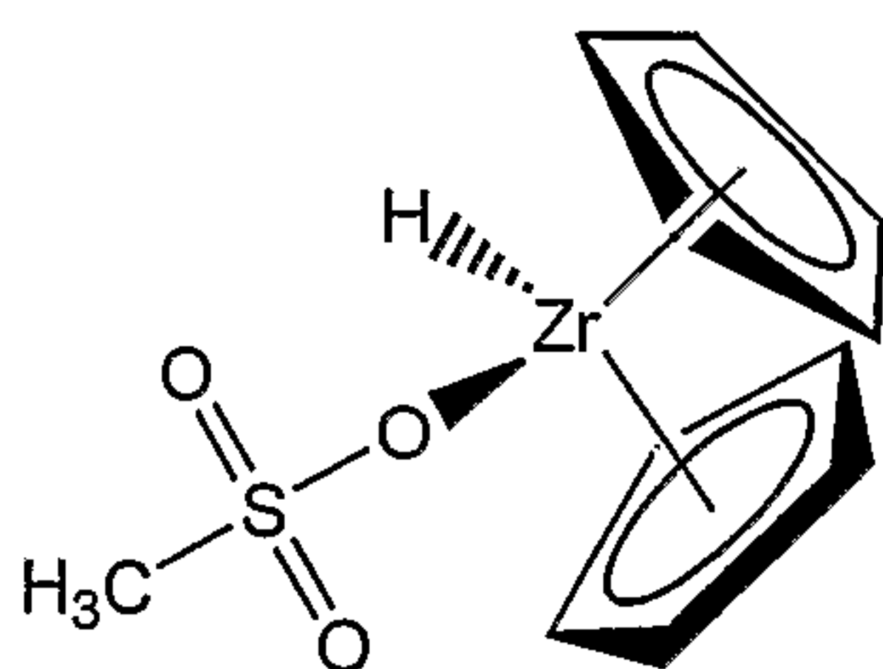
Bis(cyclopentadienyl) zirconium methylsulfonate hydride
