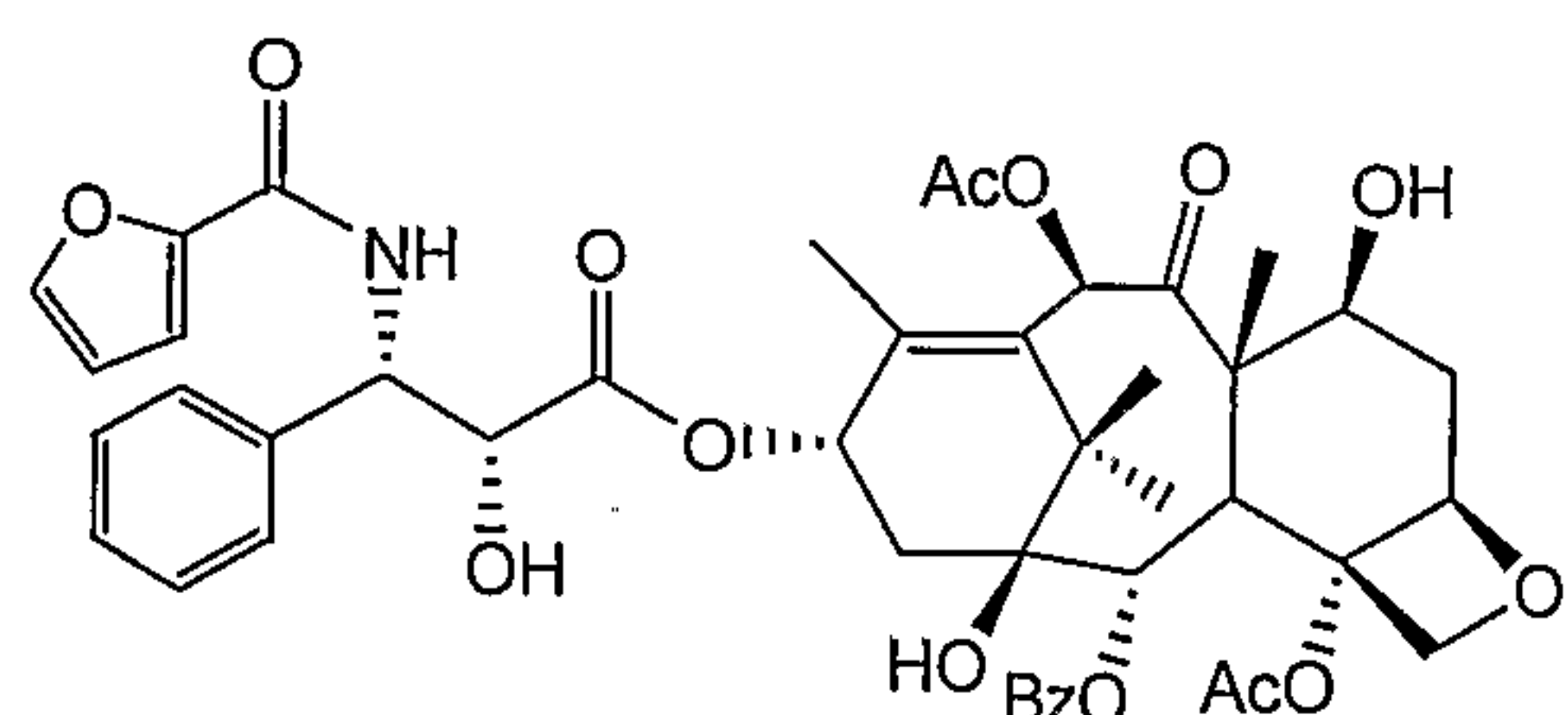
Taxol G
