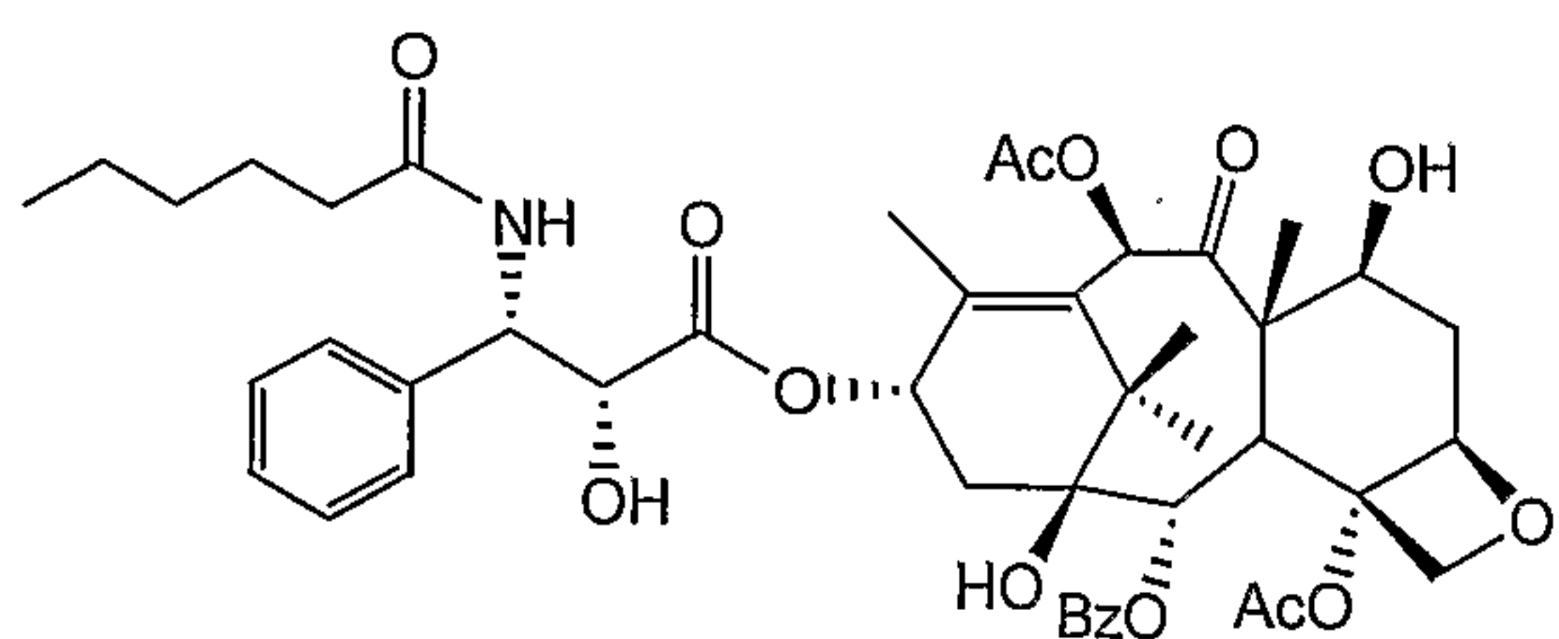
Taxol C
