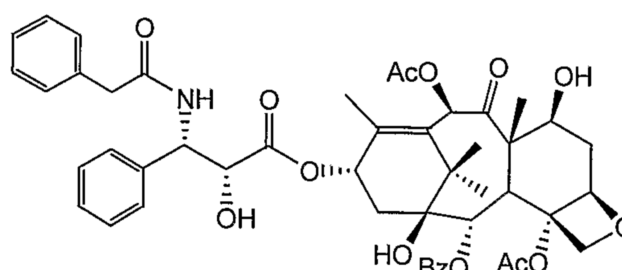
Taxol F
