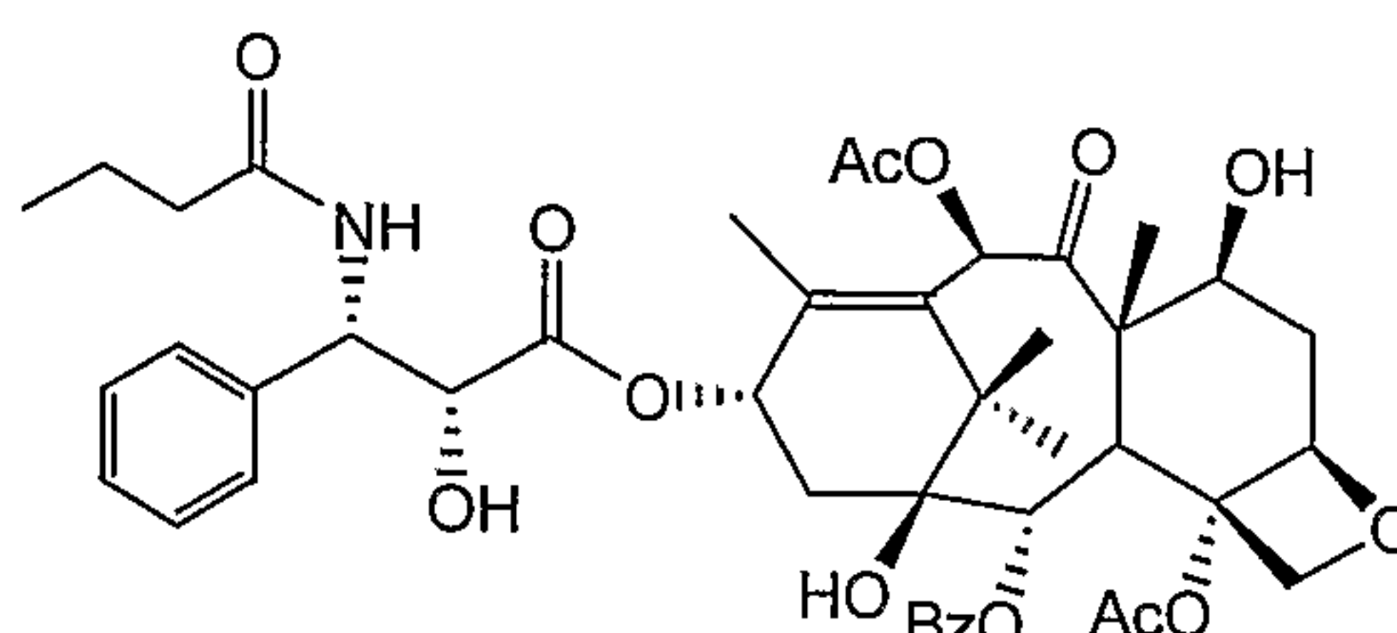
Taxol D
