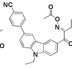
化合物113
