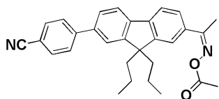
化合物38
