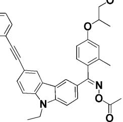
化合物138
