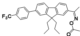
化合物55
