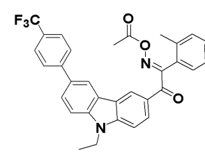
化合物132
