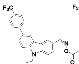
化合物120
