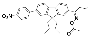
化合物6
