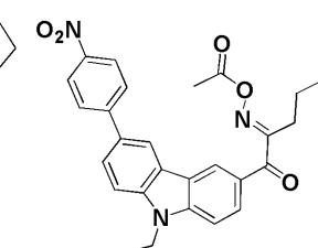
化合物85
