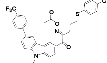
化合物136
