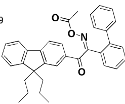
PI-12
