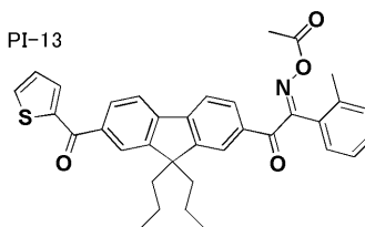
PI-16
