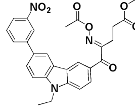
化合物100
