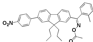
化合物7
