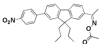
化合物4
