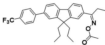
化合物56
