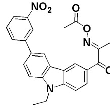
化合物96
