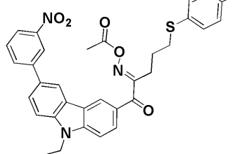
化合物102
