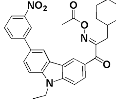
化合物102
