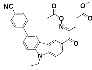
化合物117
