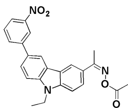
化合物90
