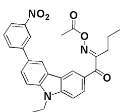
化合物101
