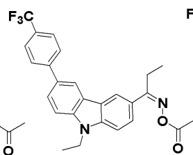
化合物121
