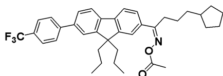
化合物61
