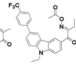
化合物130
