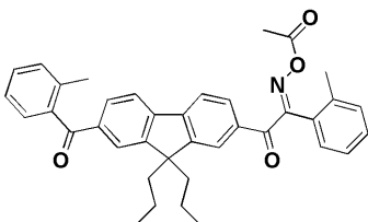
PI-14
