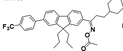
化合物59
