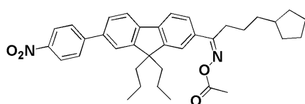
化合物10
