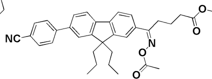
化合物40
