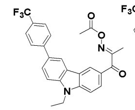
化合物129
