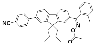
化合物41
