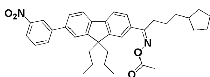
化合物27
