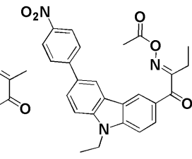
化合物79
