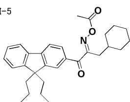
PI-6
