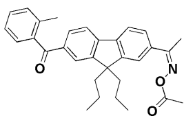
PI-4
