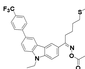
化合物127
