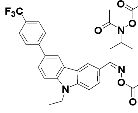
化合物128
