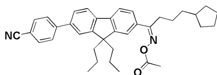
化合物44
