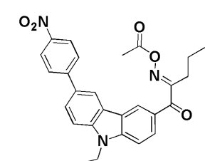
化合物80
