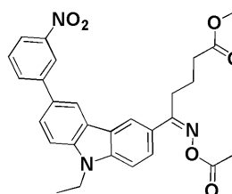
化合物91
