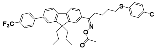
化合物59
