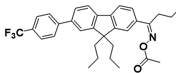
化合物57
