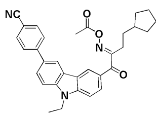
化合物118
