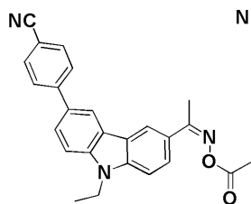
化合物107
