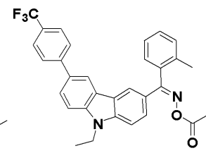
化合物126
