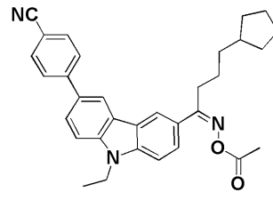
化合物113
