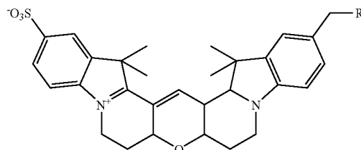
Cy3B
