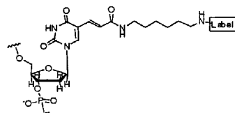
L 2 Linker:
