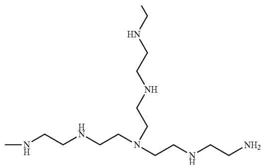
PEI: Polyethyleneimine
