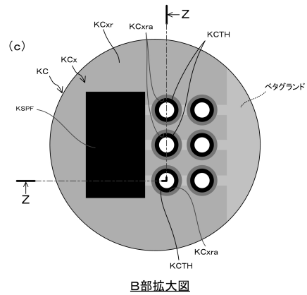
B部拡大図
