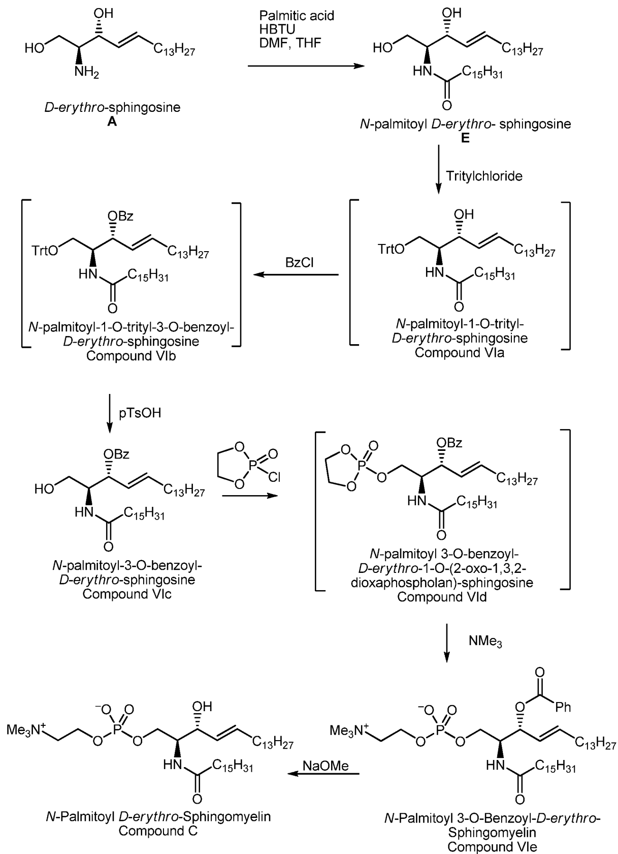
Scheme VI
