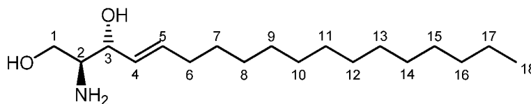
D-erythro-sphingosine
