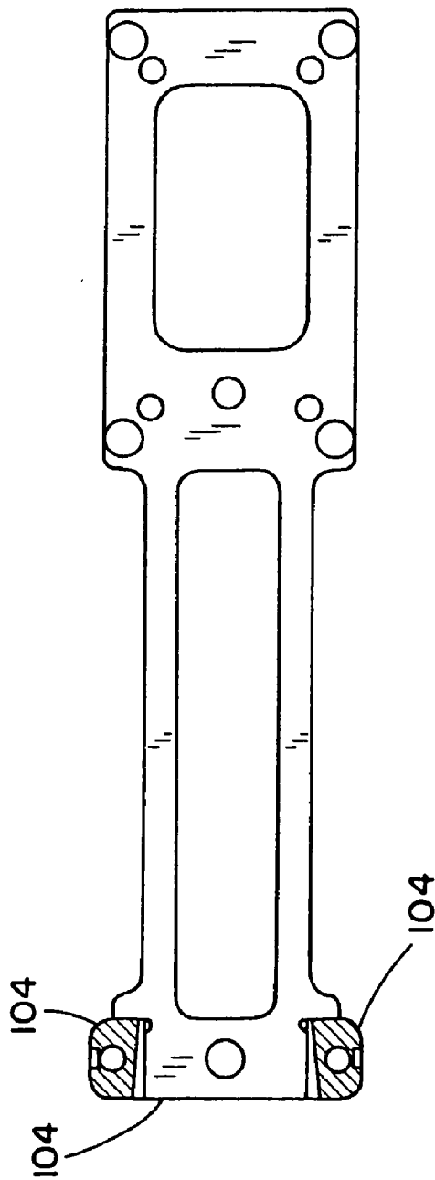
Section A-A FIG. 9b
