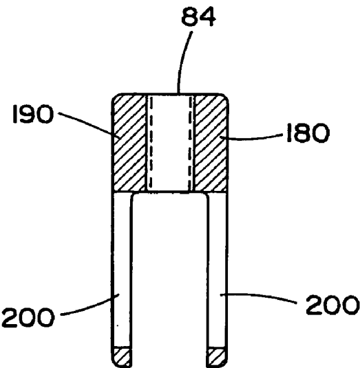
Section A-A FIG. 11c
