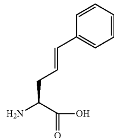
Styryl-Ala
