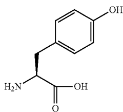
Tyr(tBu)
