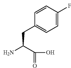
Phe(4-F)
