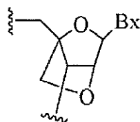
LNA ( \beta -D配置) 架橋 = 4'-CH 2 -O-2'
