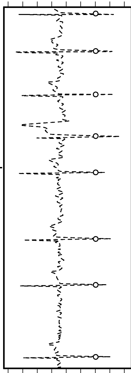
AFib Strip
