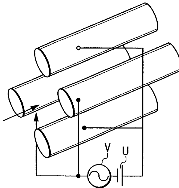
QUADRUPOLE ELECTRODE
