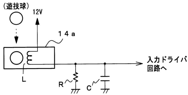
(A) 近接スイッチ（始動ロスイッチ14aの例）
