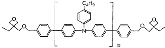
화합물 4
