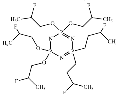
Hexakis(2-fluoropropoxy)phosphazene
