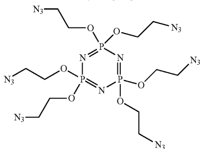
2,2,4,4,6,6-hexakis(2-azidoethoxy)-1,3,5,2λ5,4λ5,6λ5-triazatriphosphinine
