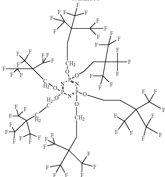
Hexakis(3,3-bis(trifluoromethyl)-4,4,4-trifluorobutoxy)phosphazene
