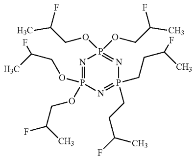
Hexakis(2-fluoropropoxy)phosphazene
