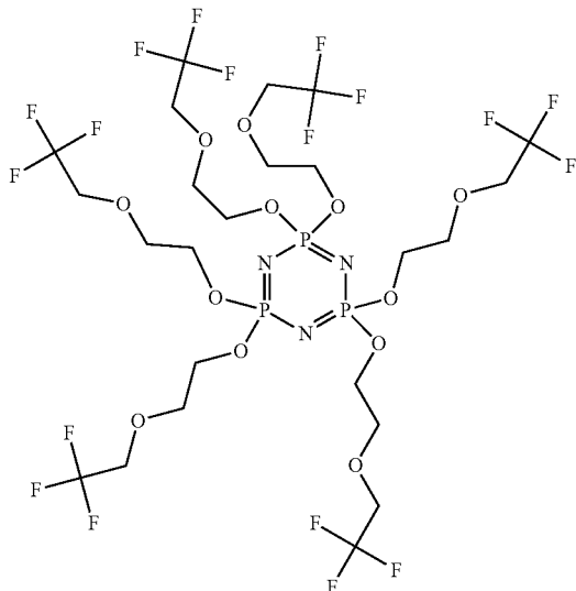
Hexakis(2-(2,2,2-Trifluoroethoxy)ethoxy)phosphazene
