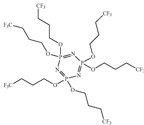
Hexakis(4,4,4-trifluorobutoxy)phosphazene
