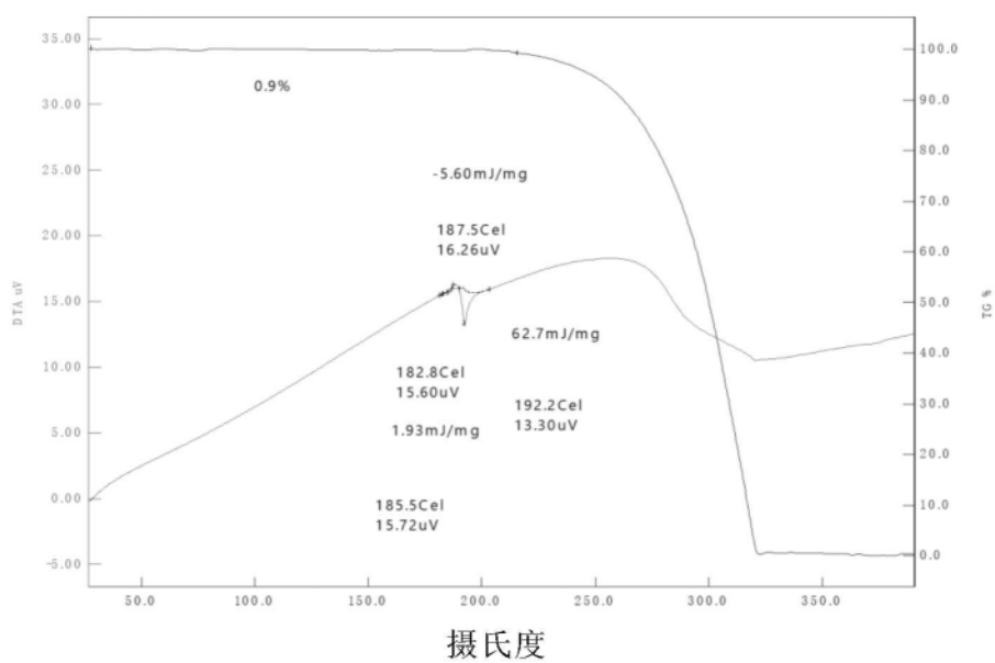
化合物 A 晶型 2 的 TG/DTA 热谱图
