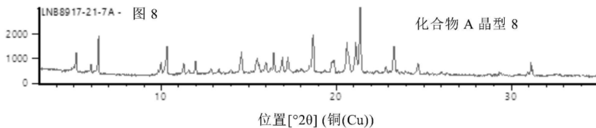
化合物 A 晶型 8 的 XRPD 衍射图
