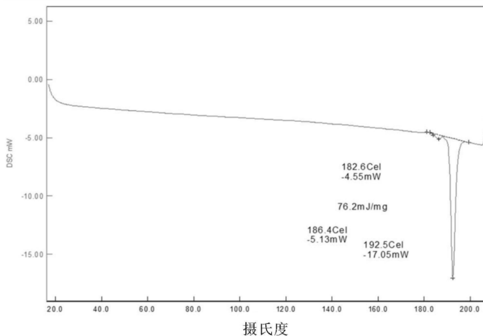
化合物 A 晶型 4 的 DSC 热谱图（第二加热循环）
