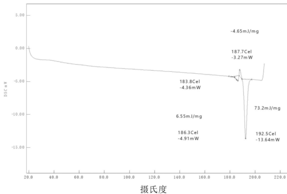
化合物 A 晶型 1 的差示扫描量热法 (DSC) 热谱图 (初始加热循环)
