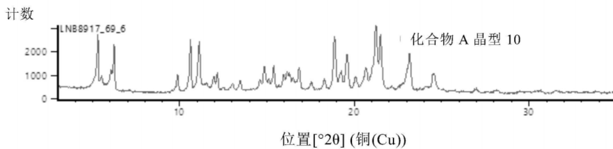
化合物 A 晶型 10 的 XRPD 衍射图
