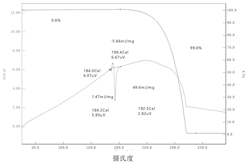
化合物 A 晶型 1 的热重分析/差热分析 (TG / DTA) 热谱图
