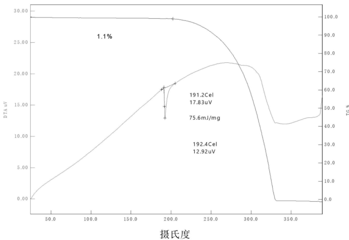
化合物 A 晶型 11 的 TG/DTA 热谱图
