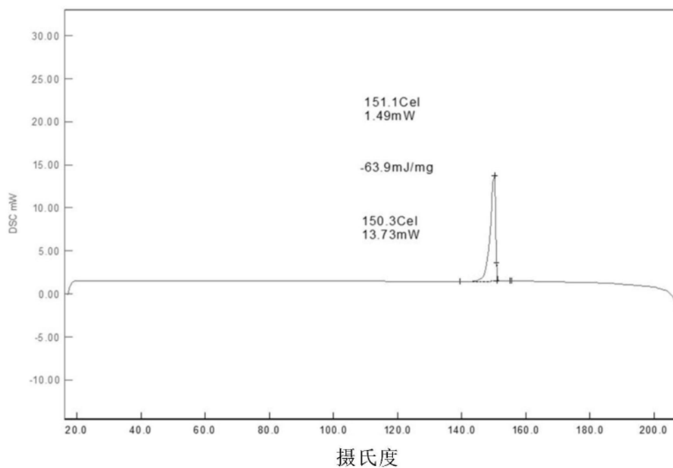
化合物 A 晶型 4 的 DSC 热谱图（冷却循环）
