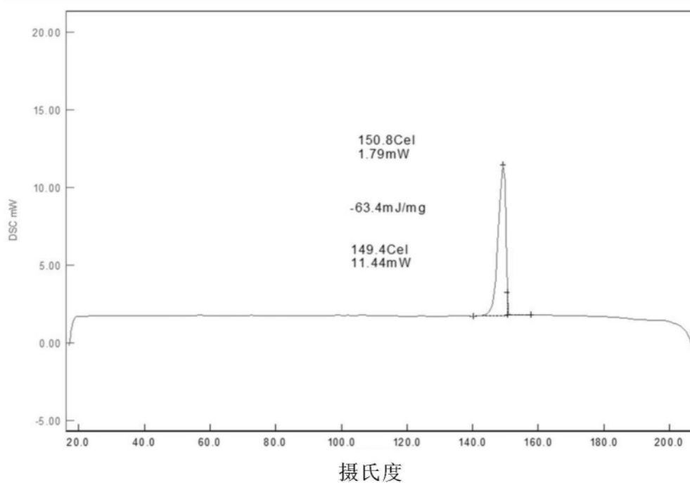
化合物 A 晶型 2 的 DSC 热谱图（冷却循环）
