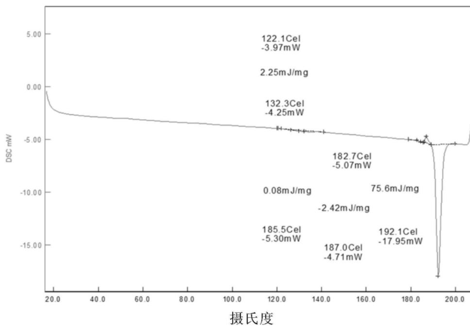
化合物 A 晶型 2 的 DSC 热谱图（初始加热循环）
