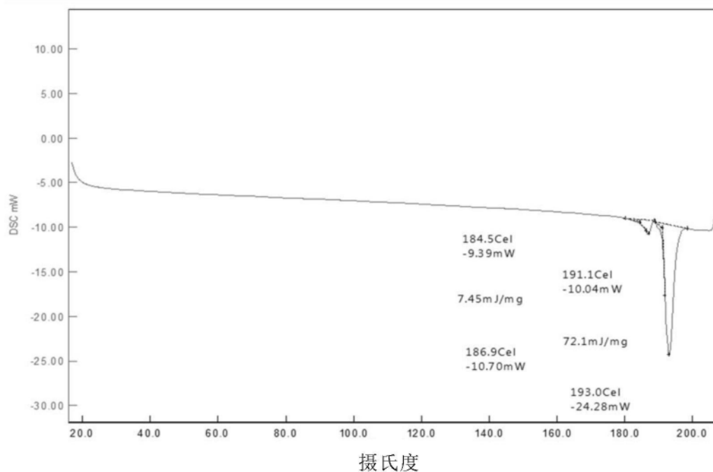
化合物 A 晶型 1 的 DSC 热谱图 (第二加热循环)
