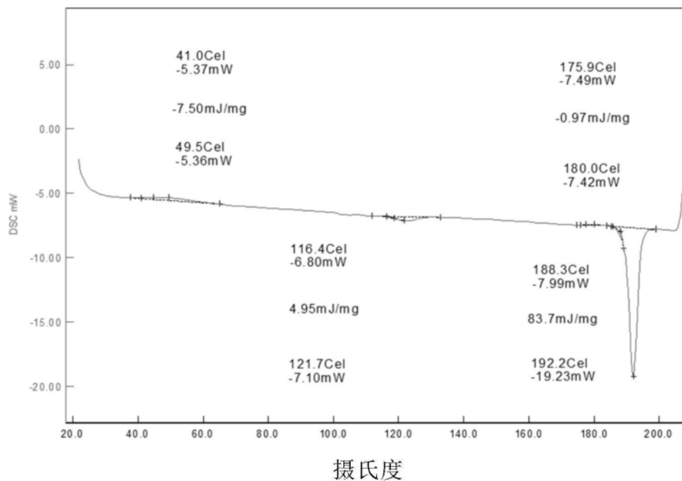
化合物 A 晶型 11 的 DSC 热谱图 (初始加热循环)
