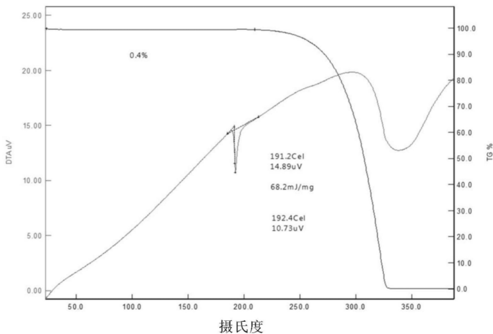
化合物 A 晶型 9 的 TG/DTA 热谱图
