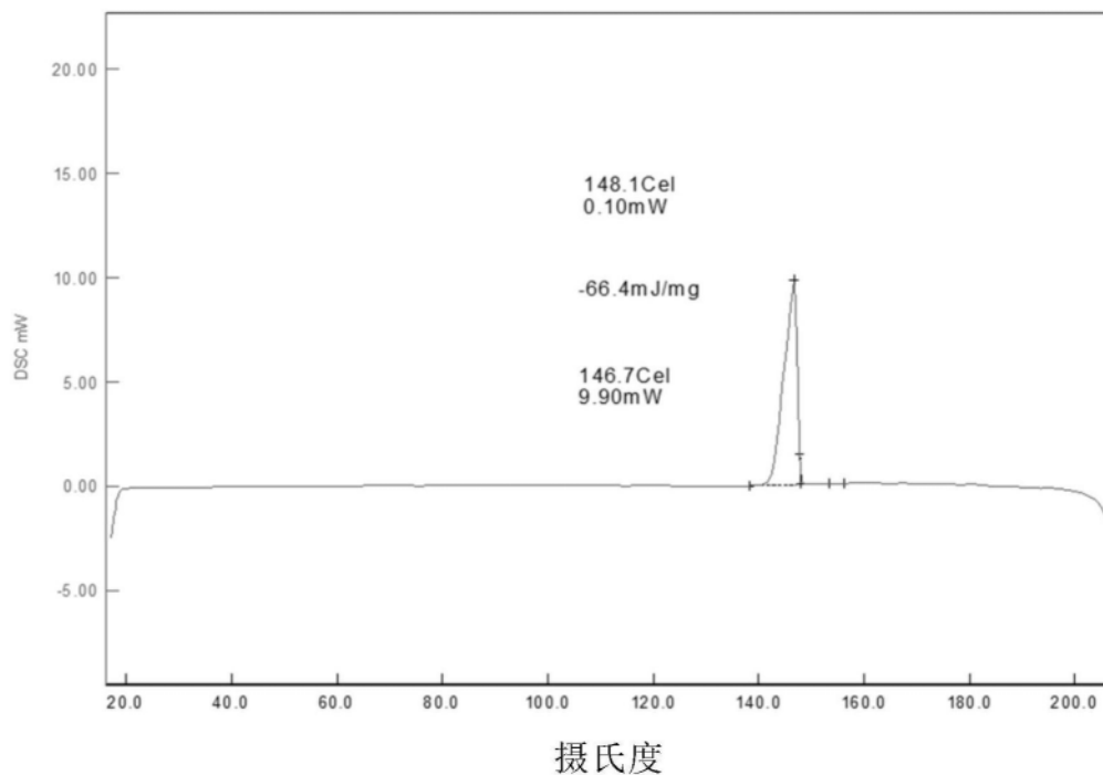
化合物 A 晶型 11 的 DSC 热谱图 (冷却循环)
