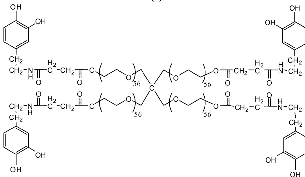
C-(PEG-DMe) 4 PEG 10K - (DMe) 4
