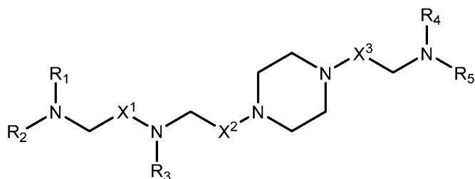
(Ia1),
