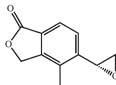
4-methyl-5-[(2R)-oxiran-2-yl]-2-benzofuran-1(3H)-one
