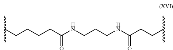
(XVI)
