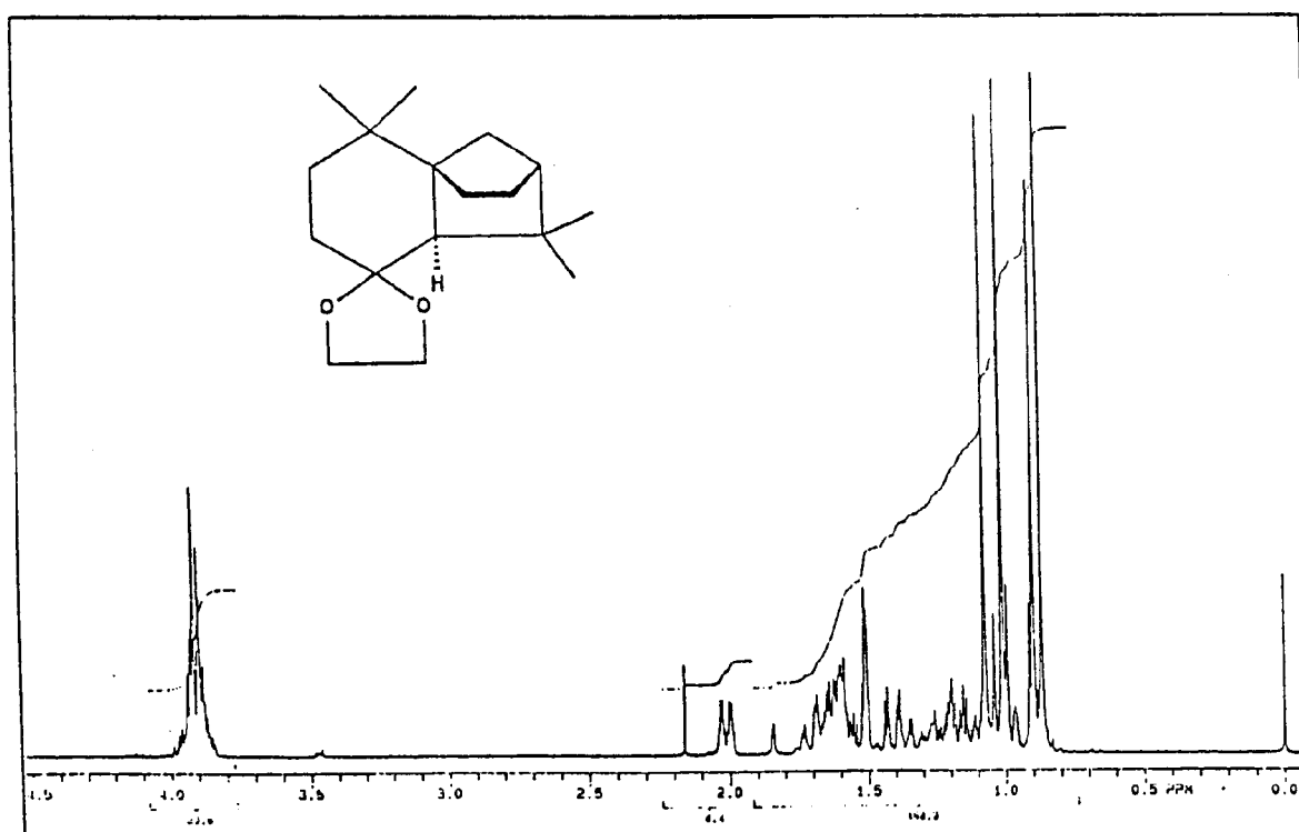
Abb. 2: ^1\text{H} -NMR-Spektrum (300 MHz, \text{CDCl}_3 ) von 5b
