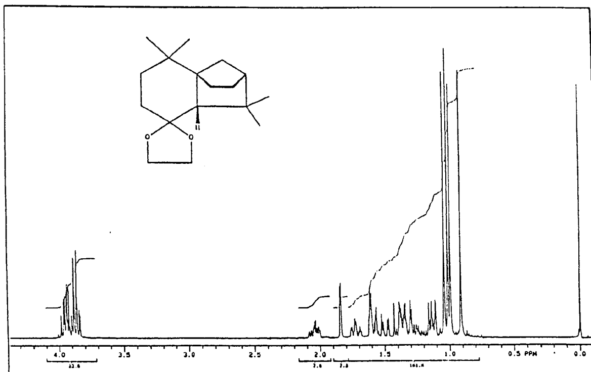
Abb. 1: ^1\text{H} -NMR-Spektrum (300 MHz, \text{CDCl}_3 ) von 5a
