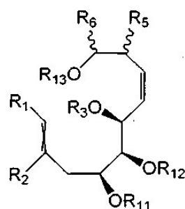
isômero \beta
