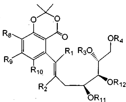
Fórmula (VI):
