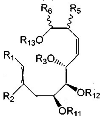
isômero \alpha
