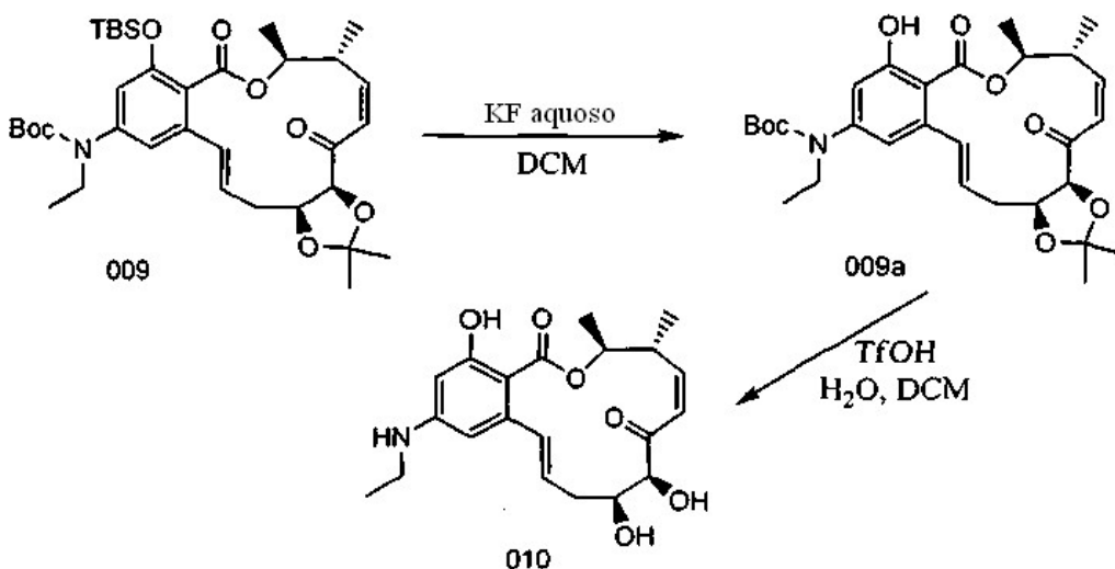
Esquema 18: Desproteção
