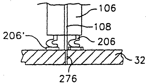
FIG. 14a
