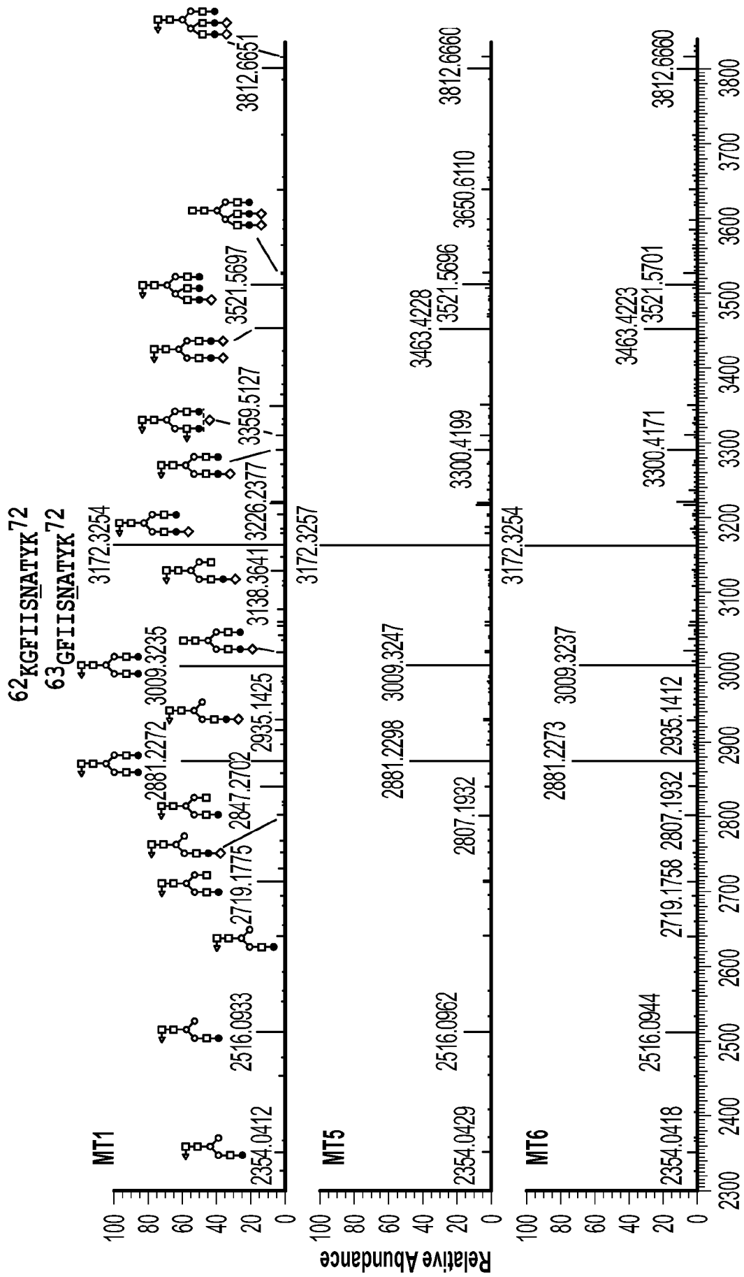
m/z FIG. 52
