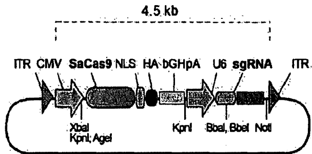
AAV-Sa-Cas9 vector: CMV-SaCas9-NLS-HA-U6-sgRNA
