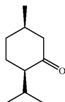
(+) - Isomenthone
