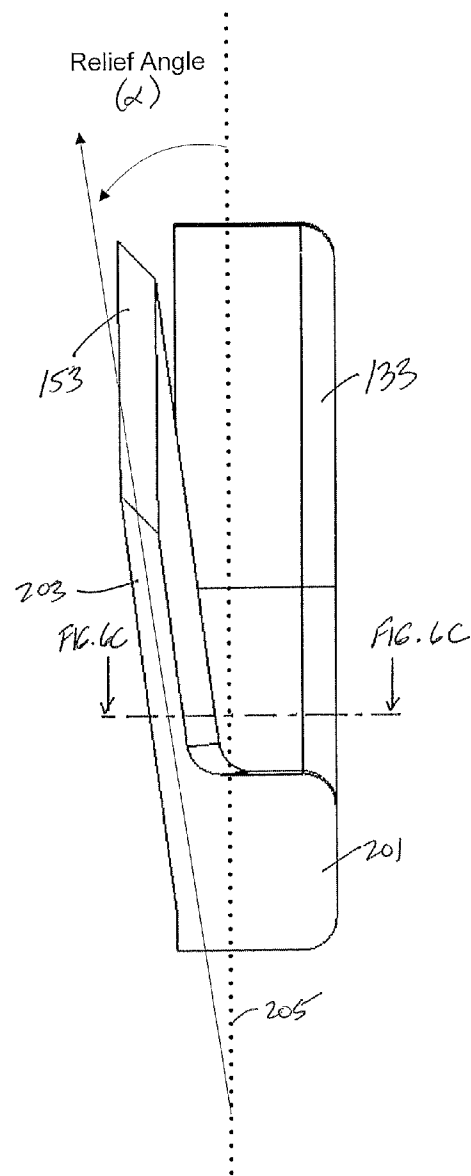
FIG. 6B
