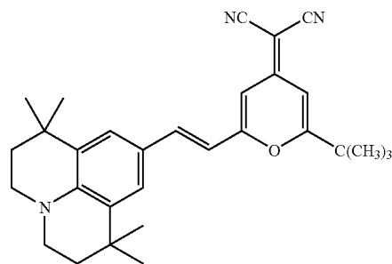
DCJTB
