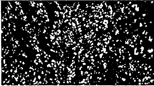
a. Compozit funcționalizat prin depunere de film polimeric pe bază de matrice chitosan cu masă moleculară mică și microparticule de Cu
