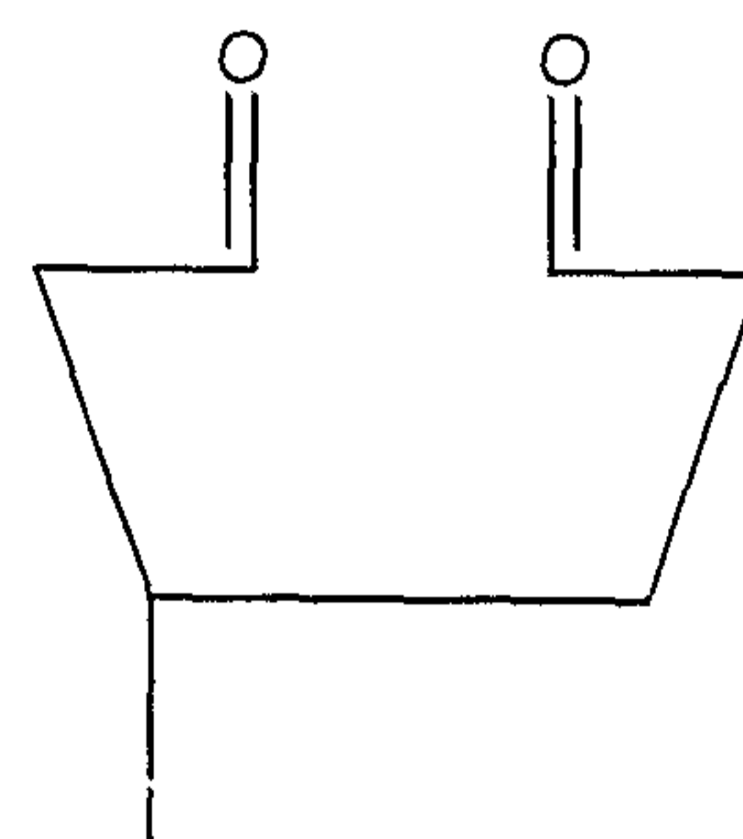
VIIc
