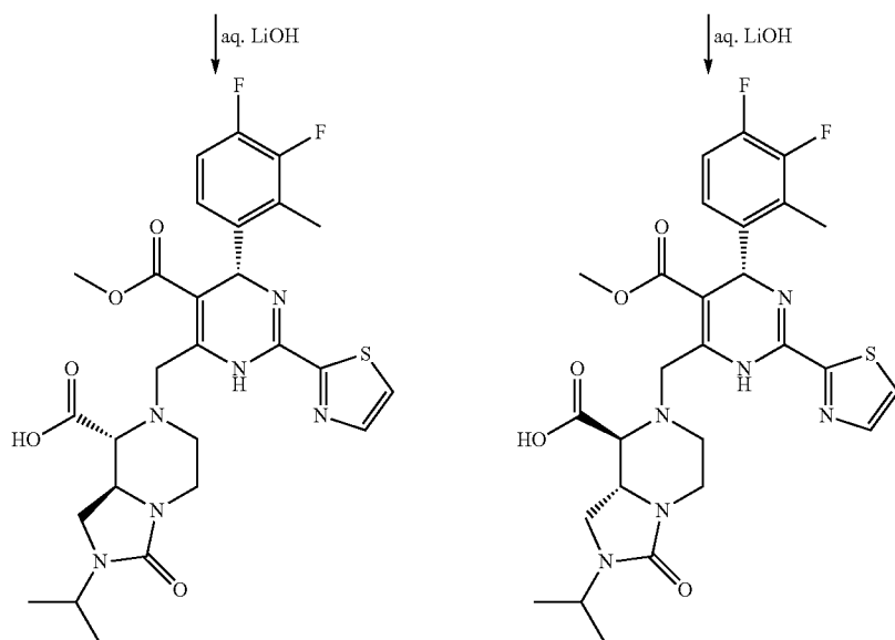
85A &amp; 85B
