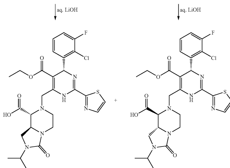
84A &amp; 84B
