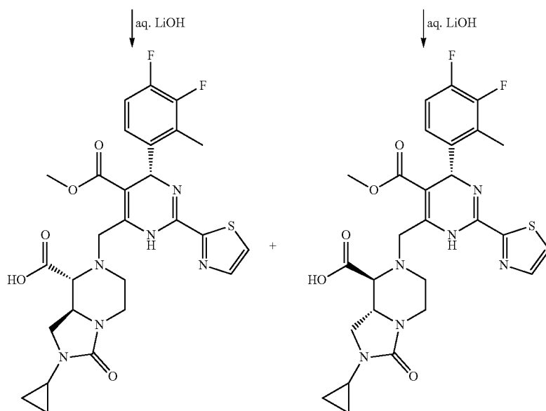
83A &amp; 83B
