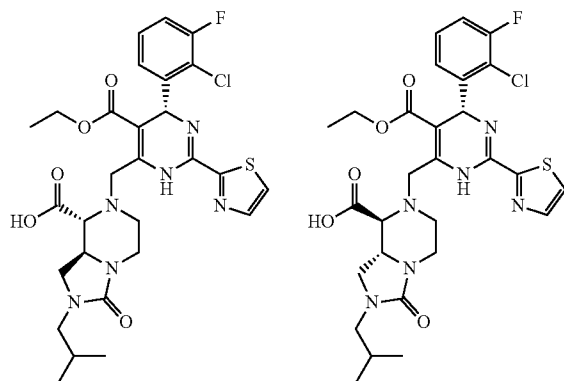
101A-1 &amp; 101B
