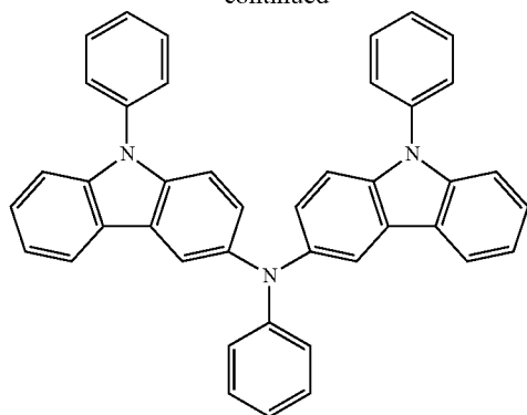
PCzPCA1
