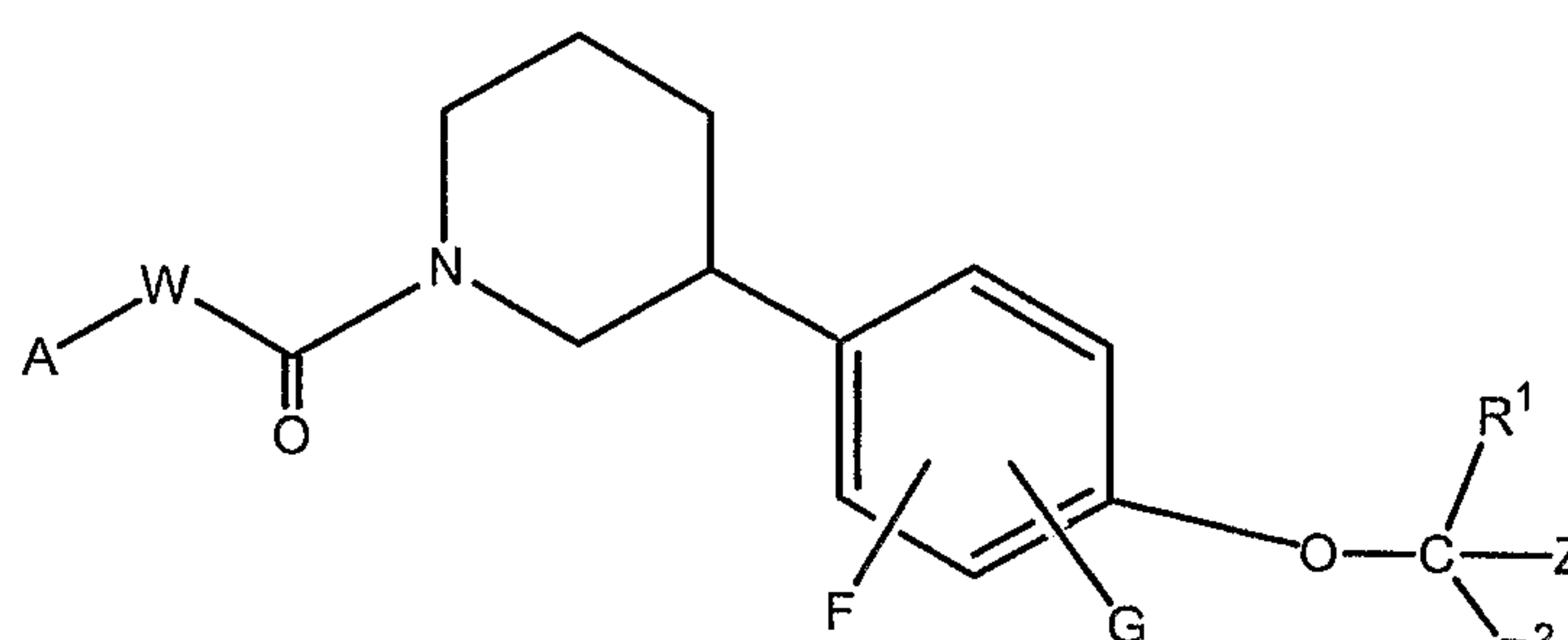
I-C
