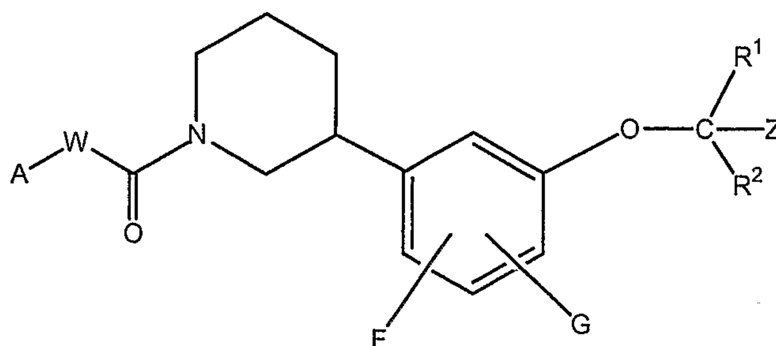
I-A
