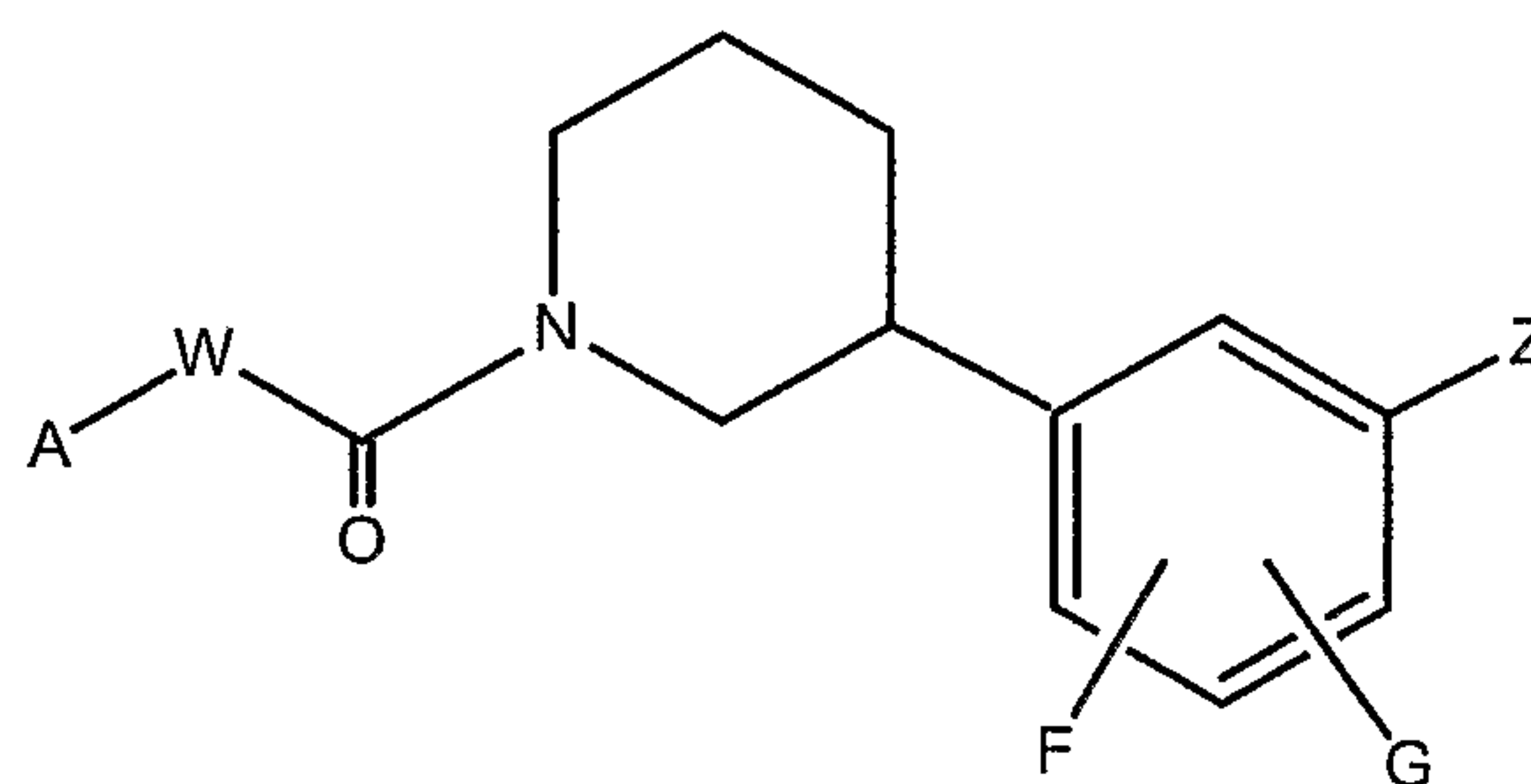
I-B
