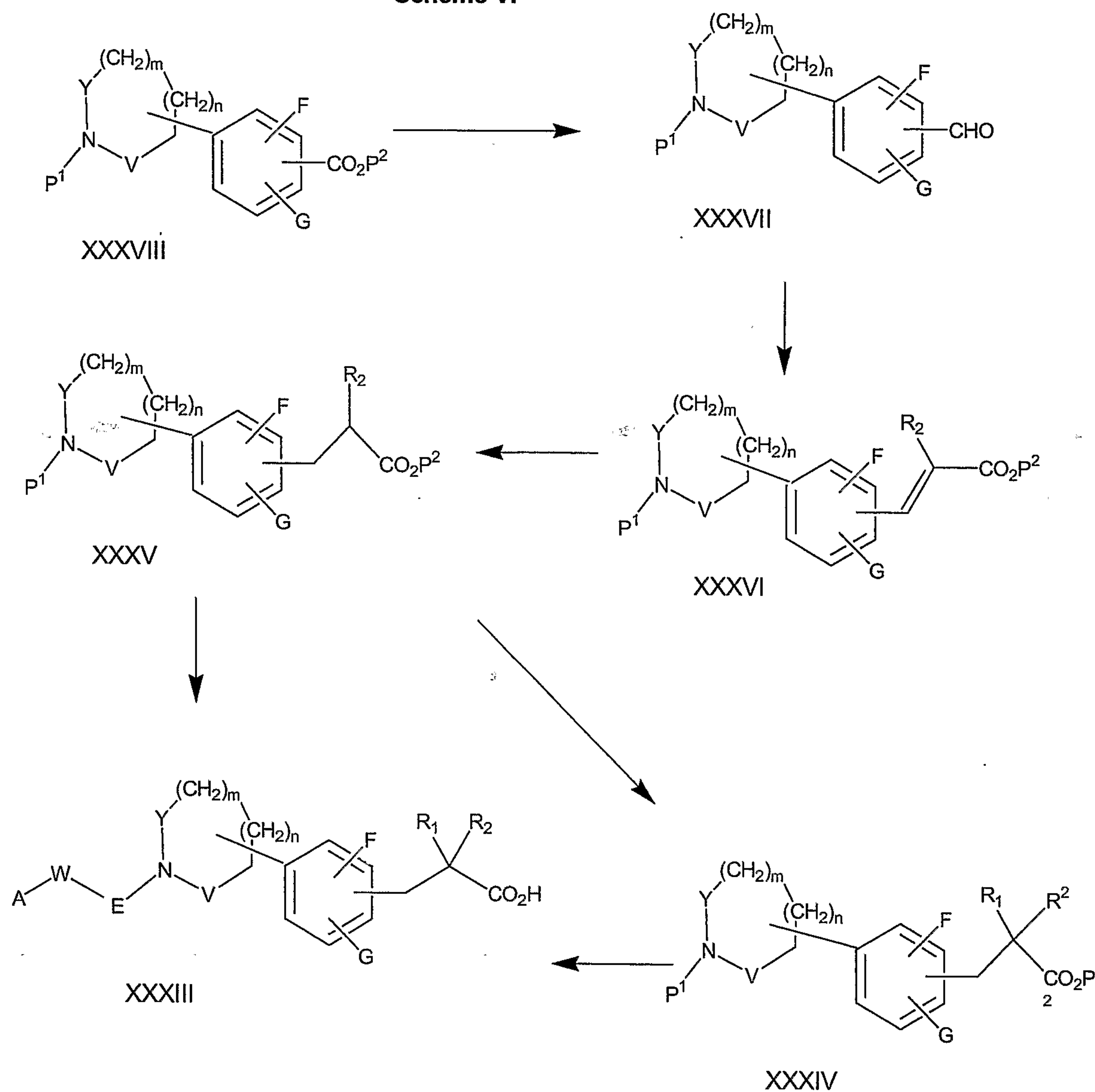
Scheme VI
