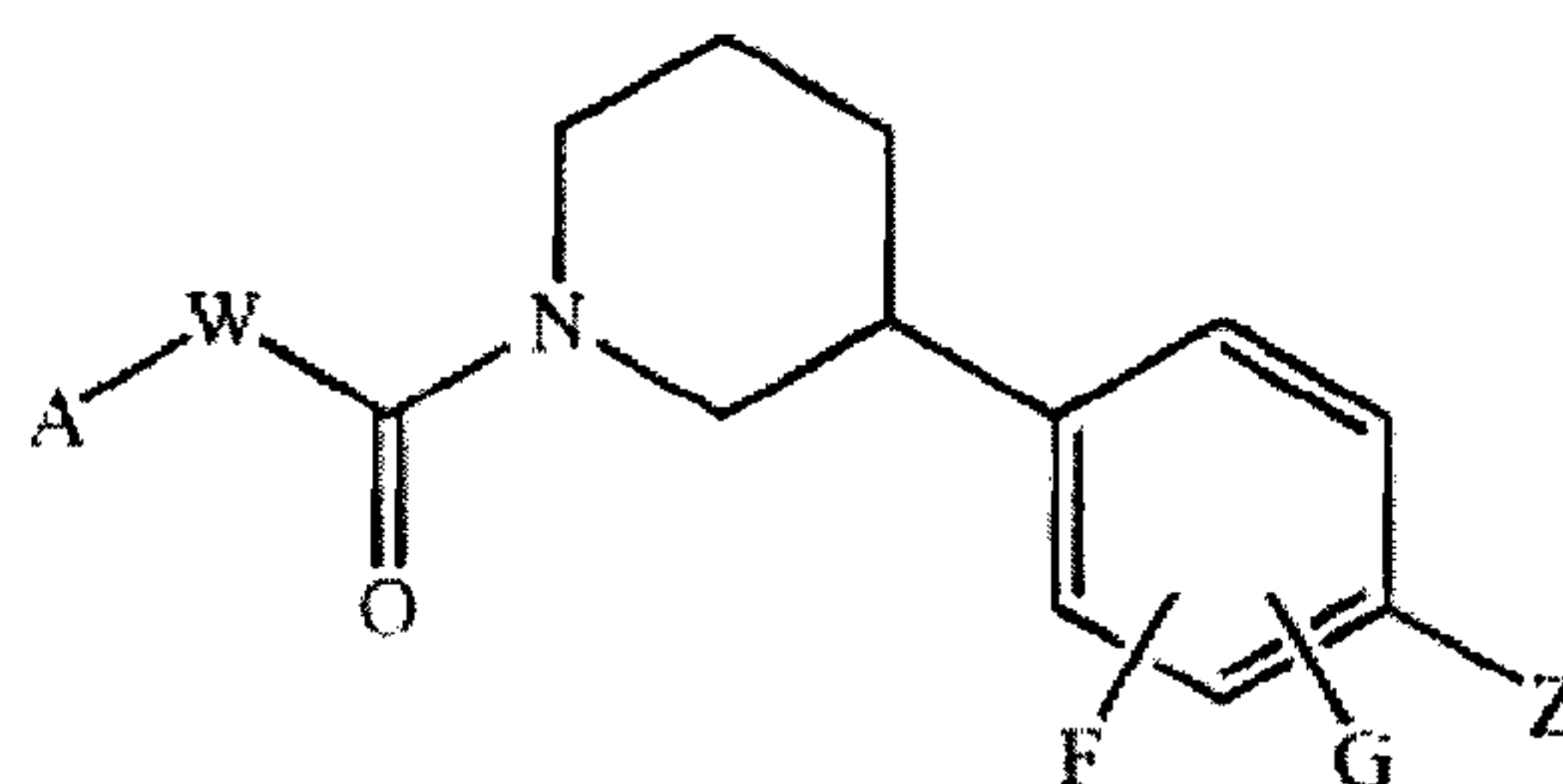
I-D
