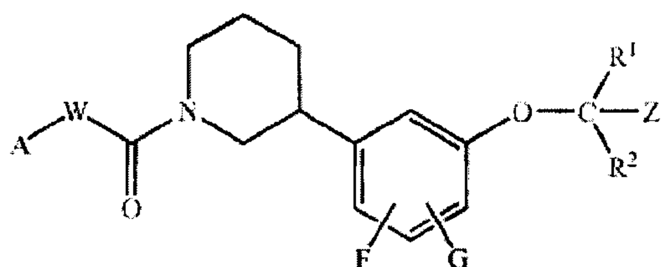
I-A
