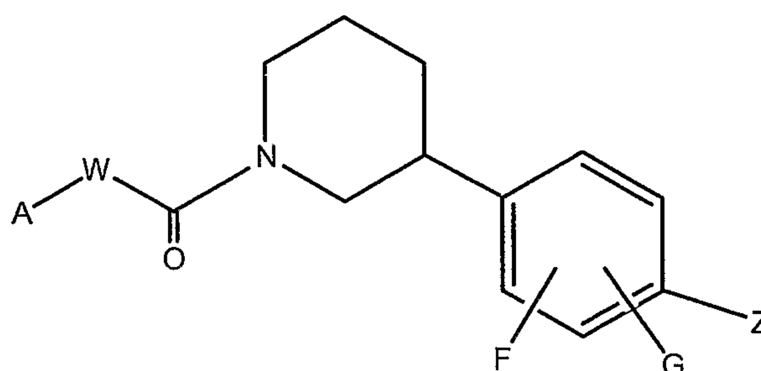
I-D
