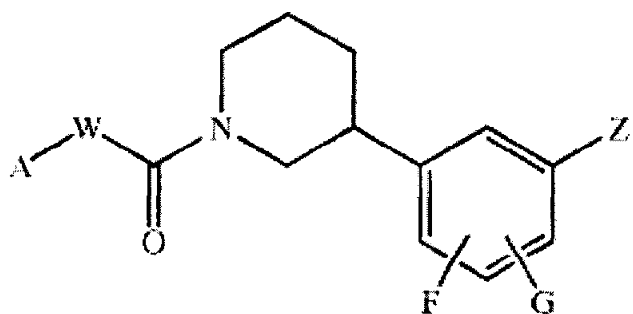
I-B
