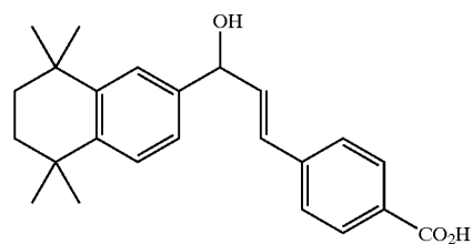
CD 666
