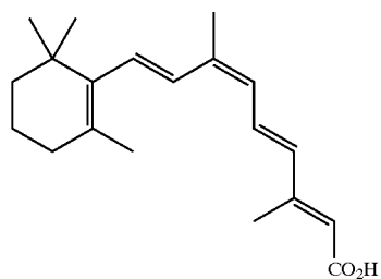
9-cis-RA
