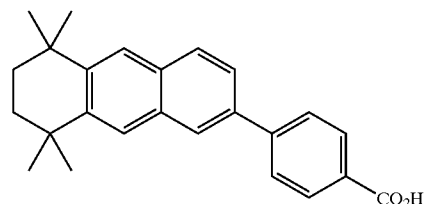
CD 367
