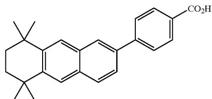
TTAB
