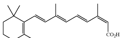
13-cis-RA
