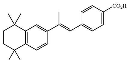
TTNPB
