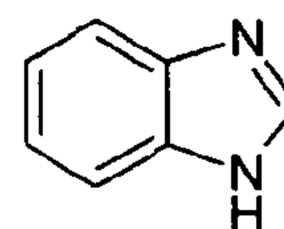
benzoimidazole
