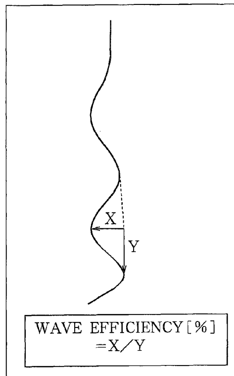
FIG. 26
