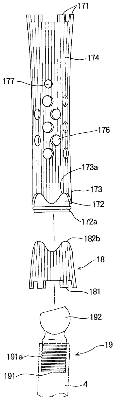
FIG. 30
