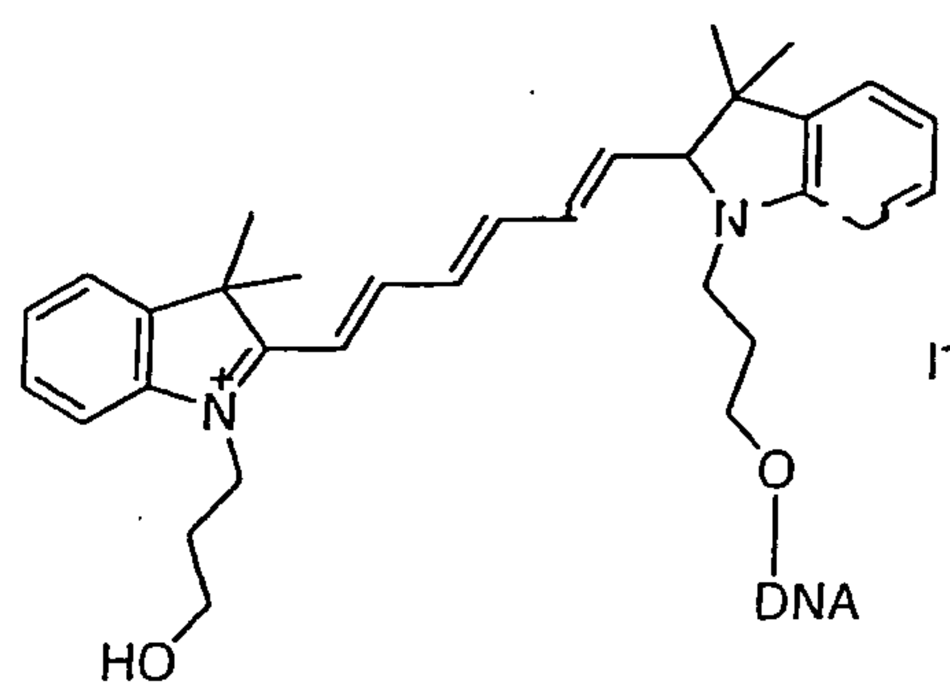
ODN-4
