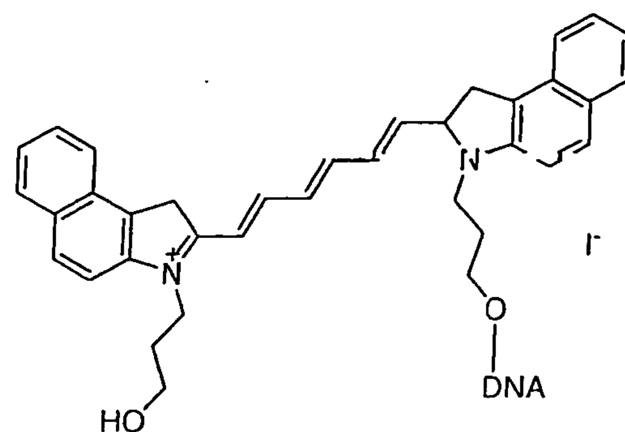
ODN-5
