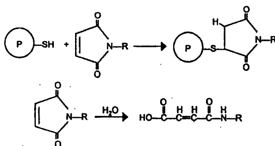
马来酰亚胺反应式
