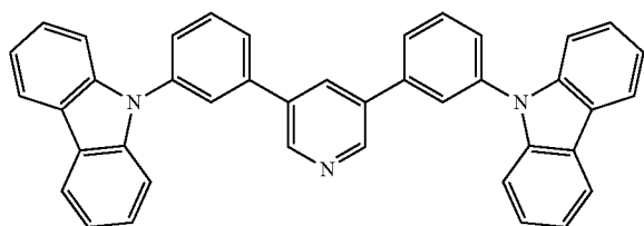
(vii) 3,5DCzPPy
