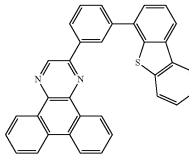
(iii) 2mDBTPDBq-II
