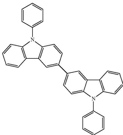
(viii) PCCP
