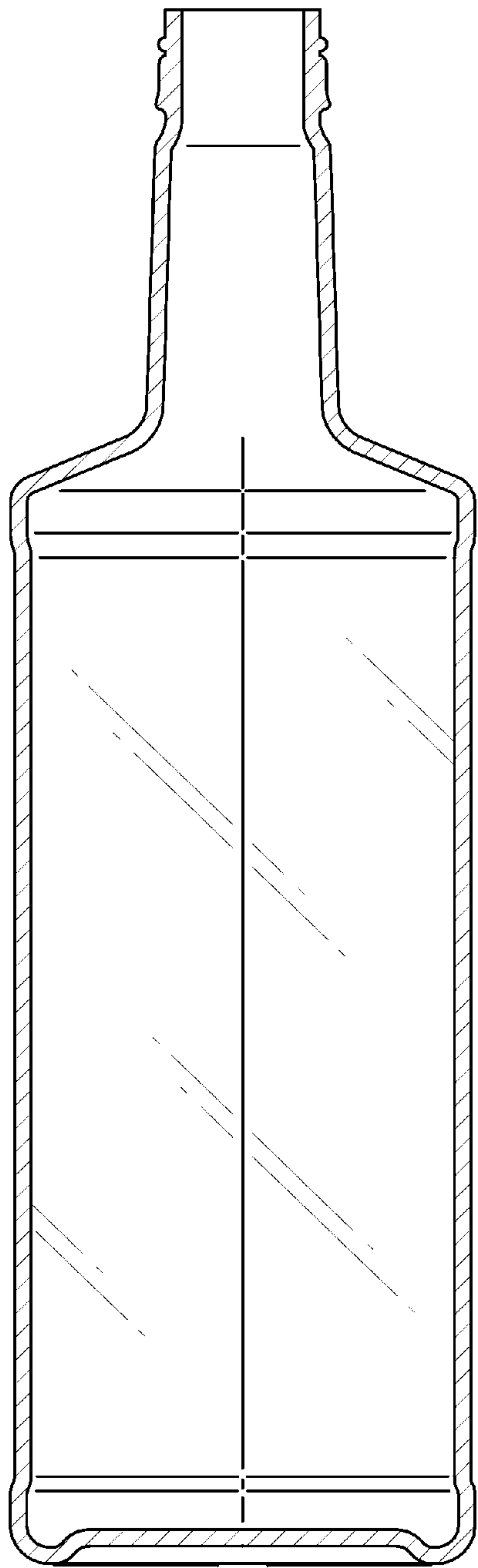
【B-B 剖面圖】
