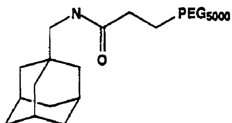
Ad-PEG 5000
