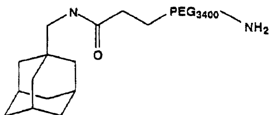
Ad-PEG 3400
