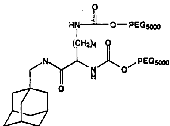
Ad-(PEG 5000 ) 2
