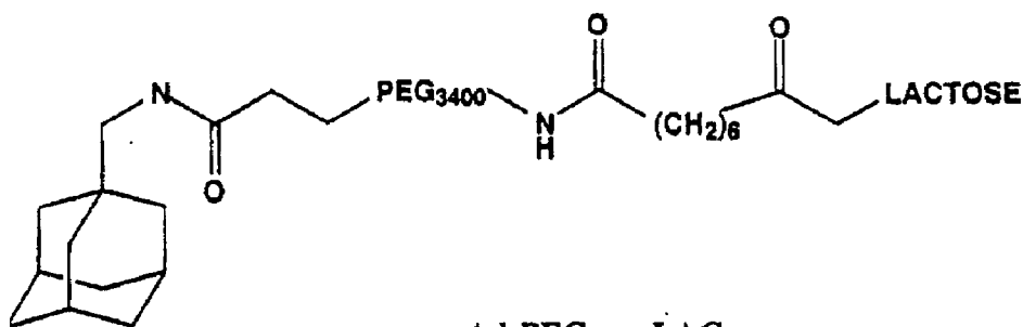
Ad-PEG 3400 -LAC
