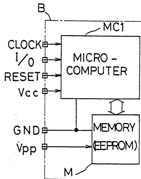
FIG. 4. IC CARD
