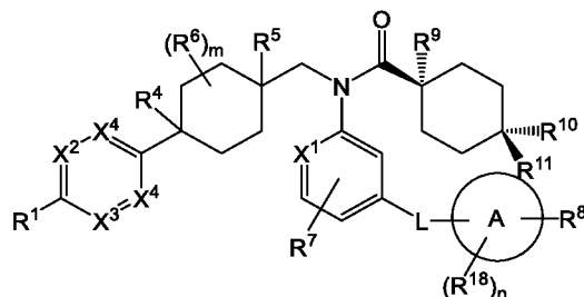
Formula (Ia).
