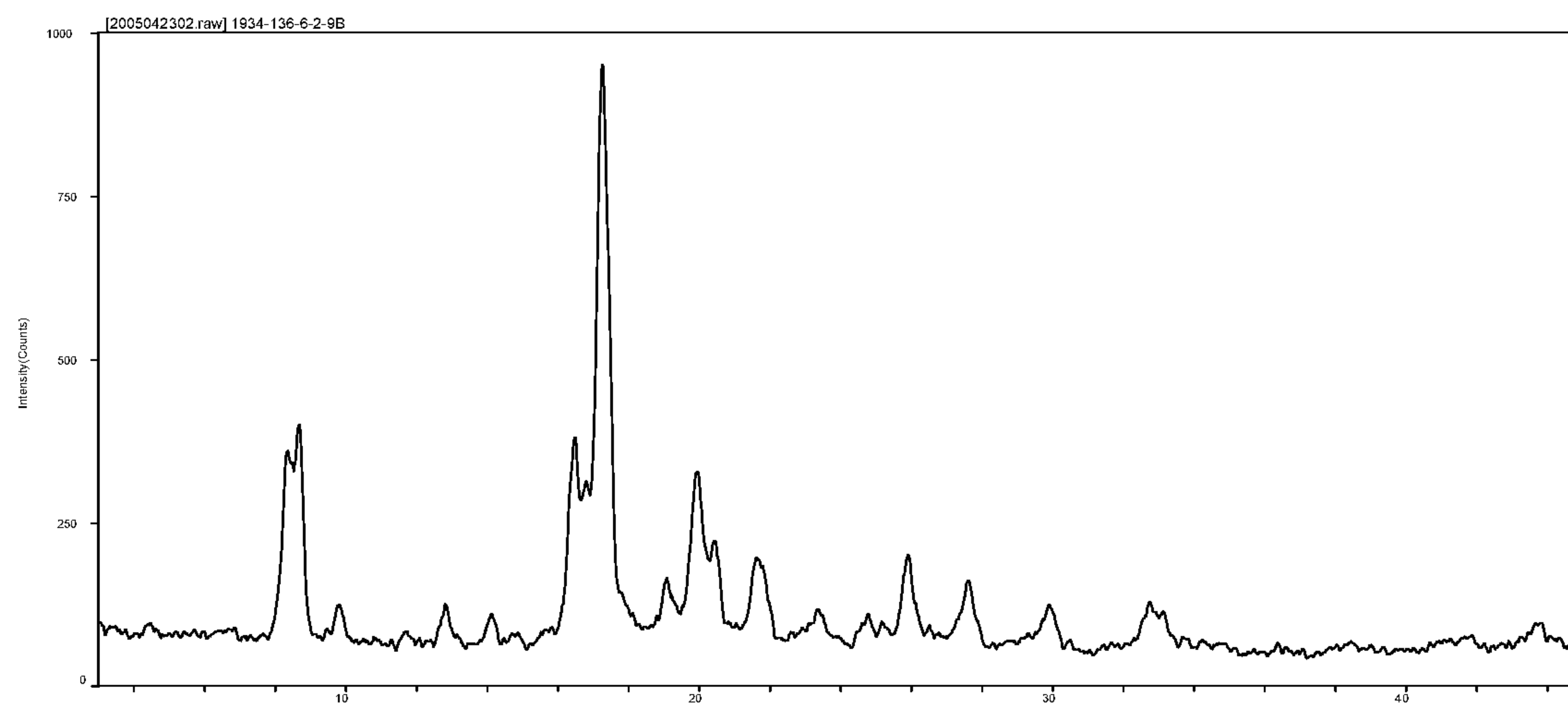
FIG. 11 XRPD Form Va
