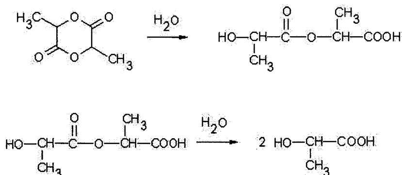
Schema 2. Reaktionsschema der Dilactidhydrolyse
