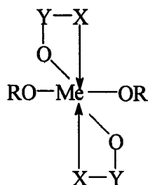
Schema 3. Allgemeine Struktur der zur Polykondensation von L-, D- bzw. D,L-Milchsäure sowie den Estern dieser Milchsäuren vorgeschlagenen Chelate von Metallen der IV. Nebengruppe
